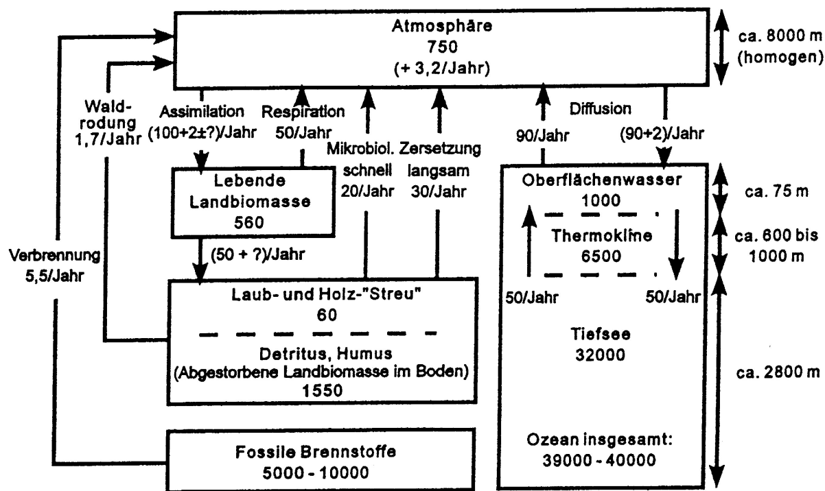
Abb. 4: \text{CO}_2 -Austausch zwischen Atmosphäre, Biosphäre und Ozean – Inventar in Gt C, Flüsse in Gt C/a (ROEDEL 2000).
