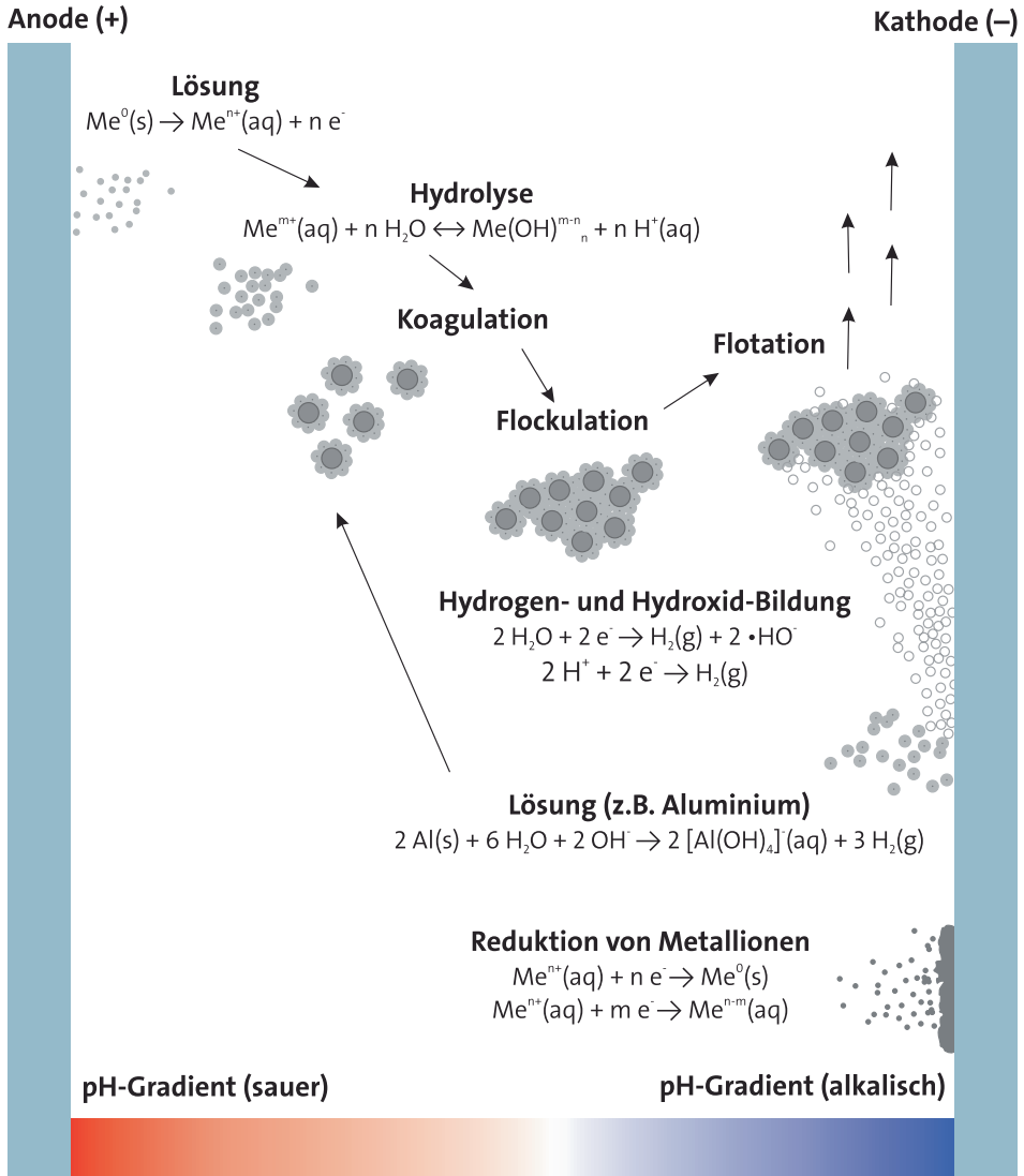
Abb. 3.12 Prinzip der Elektrokoagulation. (Verändert nach Vepsäläinen 2012)
