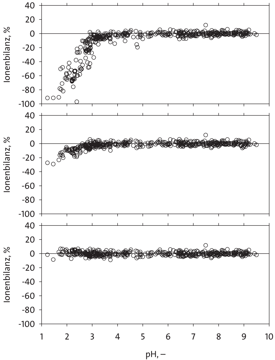
Abb. 2.4 Ionenbilanz, berechnet nach unterschiedlichen Methoden. Oben: ohne Speziierung, Mitte: ohne Speziierung, Protonen berücksichtigt, unten: mit Speziierung und Protonen (Nordstrom et al. 2009)
