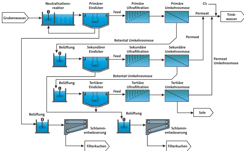
Abb. 7.8 Prinzip der Grubenwasserreinigungsanlagen eMalahleni und Kromdraai in der Provinz Gauteng/Südafrika (verändert aus Gunther und Mey 2008)
