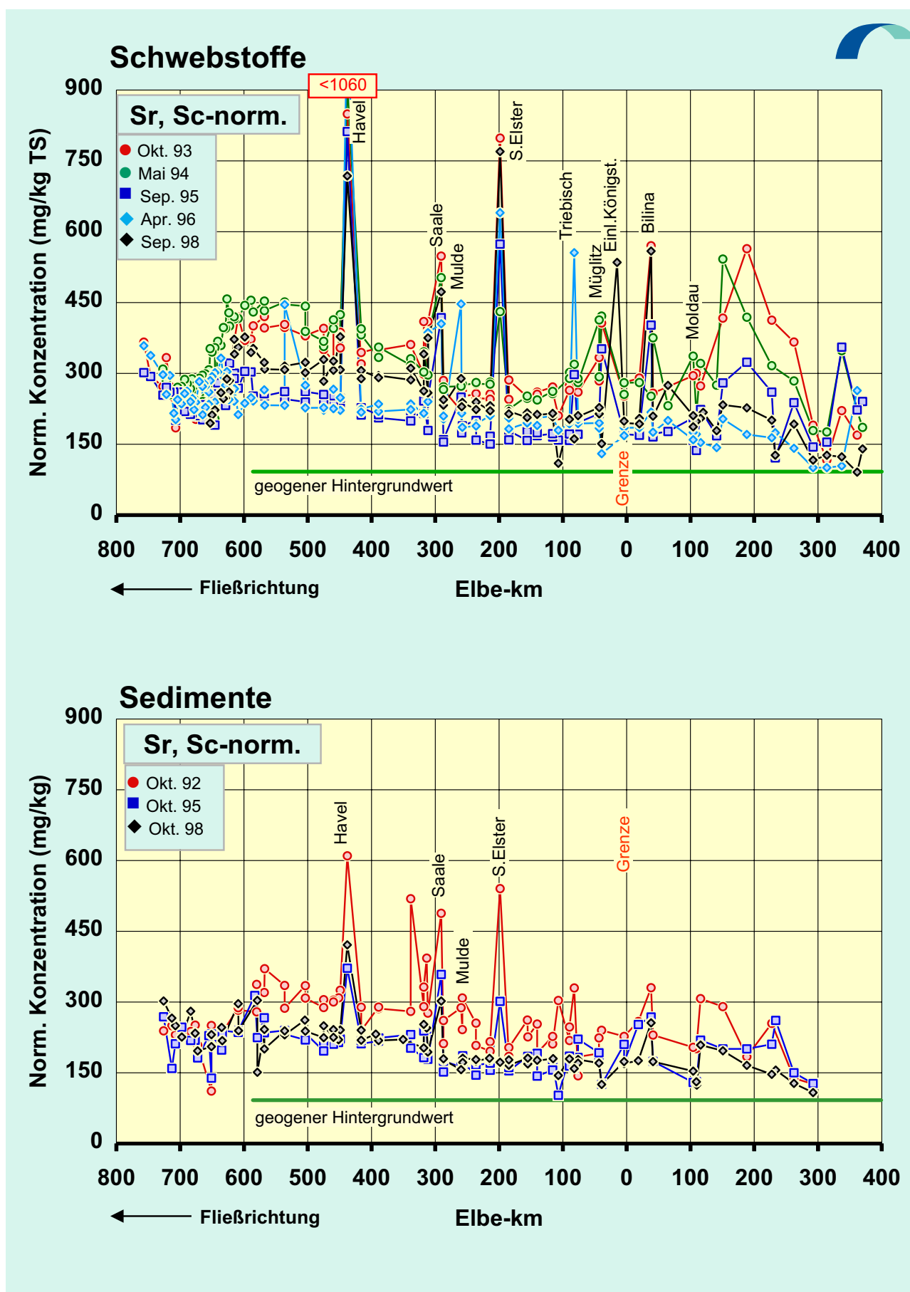
Abb.37f: Vergleich der Sc-normierten Strontium -Konzentrationen in der Schwabstoff -Trocken- substanz (TS) (oben) und der < 20-µm-Fraktion der Sedimente (unten) der Elbe von der Mündung bis zur Quelle für diverse Probenahmezeitpunkte. Normierung : C_{Sr}^{norm} = C_{Sr} / C_{Sc} \cdot C_{Sc}^0 , mit C_{Sc}^0 = 13 \text{ mg/kg}
