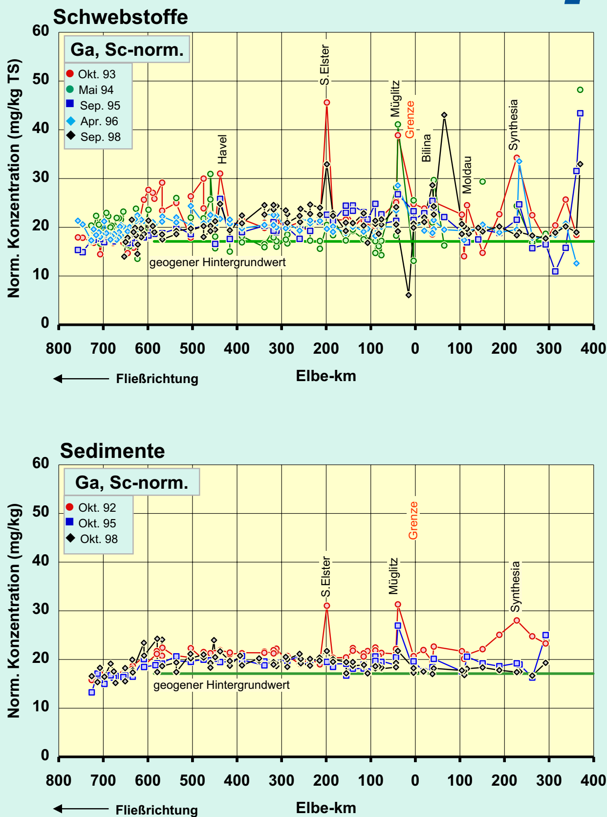
Abb.31f: Vergleich der Sc-normierten Gallium -Konzentrationen in der Schwebstoff -Trocken- substanz (TS) (oben) und der < 20-µm-Fraktion der Sedimente (unten) der Elbe von der Mündung bis zur Quelle für diverse Probennahmezeitpunkte. Normierung : C_{Ga}^{norm} = C_{Ga} / C_{Sc} \cdot C_{Sc}^0 , mit C_{Sc}^0 = 13 \text{ mg/kg}
