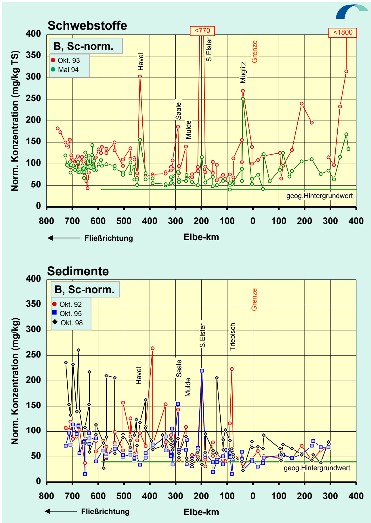
Abb.13f: Vergleich der Sc-normierten Bor -Konzentrationen in der Schwebstoff -Trockensubstanz (TS) (oben) und der < 20-µm-Fraktion der Sedimente (unten) der Elbe von der Mündung bis zur Quelle für diverse Probenahmezeitpunkte. Normierung : C_B^{norm} = C_B / C_{Sc} \cdot C_{Sc}^0 , mit C_{Sc}^0 = 13 \text{ mg/kg}
