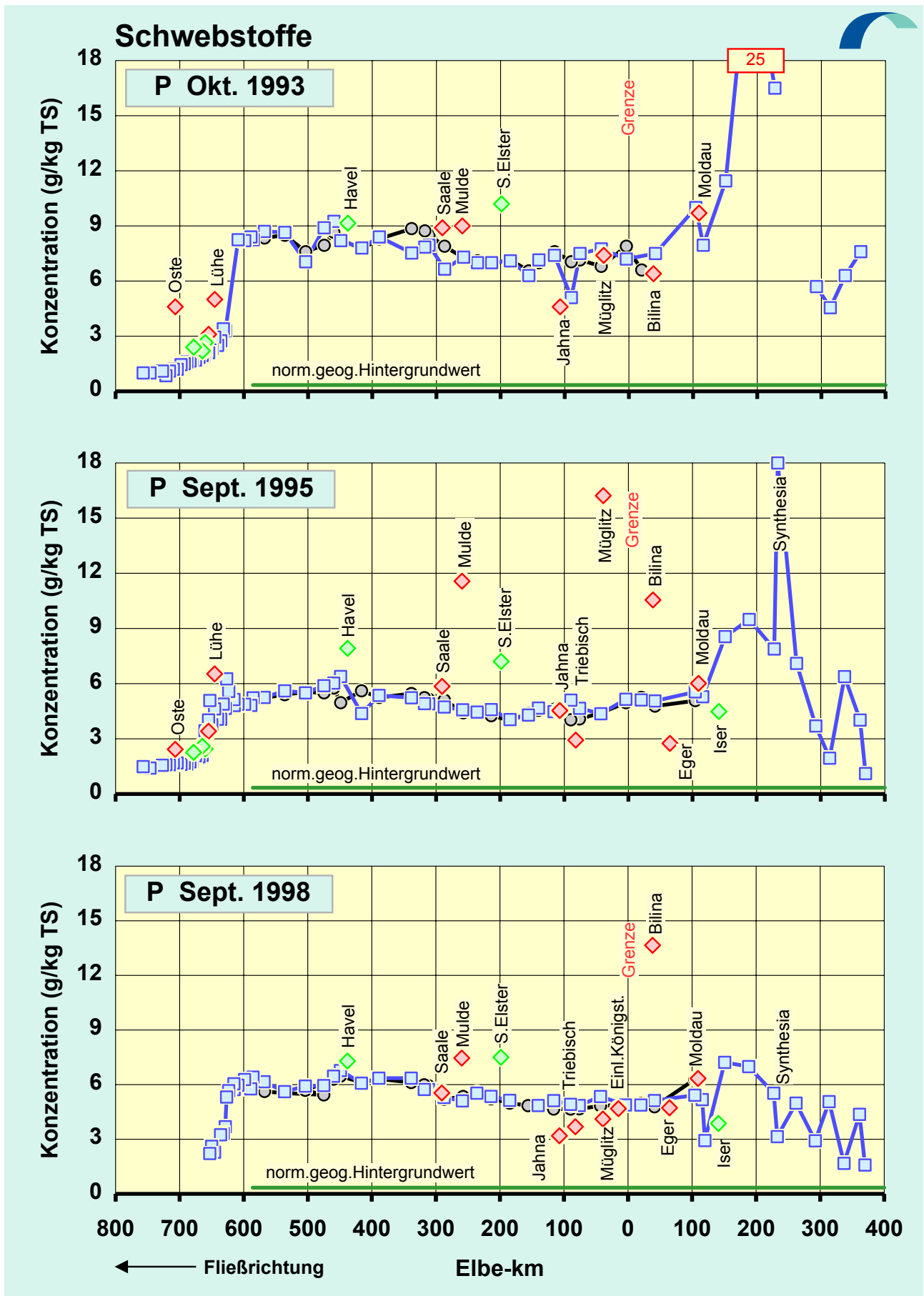
Abb.17c: Vergleich der Phosphor -Konzentrationen in der Schwebstoff -Trockensubstanz (TS) der Elbe von der Mündung bis zur Quelle: Oktober 1993 / Sept. 1995 / Sept. 1998 Legende: ■ rechtes Ufer und Flussmitte ● linkes Ufer ◆ Nebenfluss links ◆ Nebenfluss rechts
