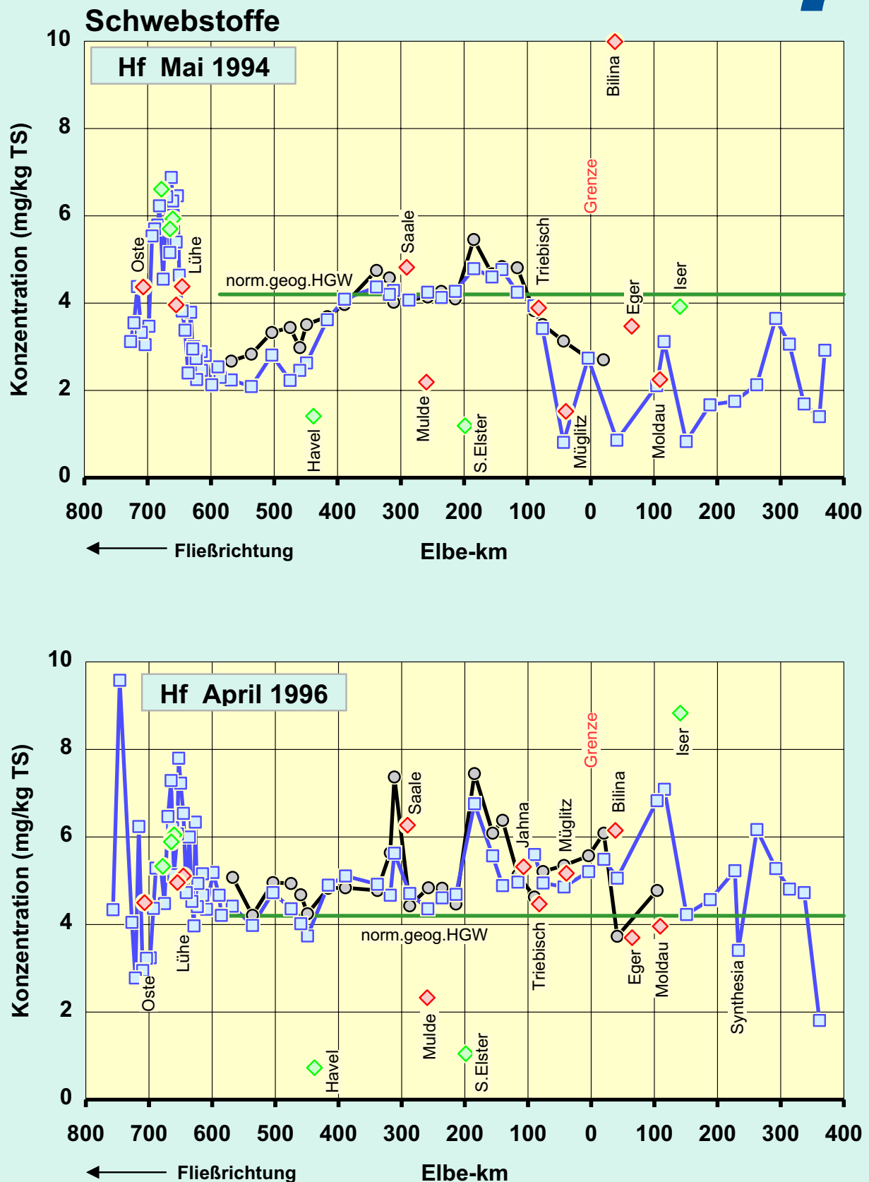
Abb.62d: Vergleich der Hafnium -Konzentrationen in der Schwebstoff -Trockensubstanz (TS) der Elbe von der Mündung bis zur Quelle: Mai 1994 / April 1996
