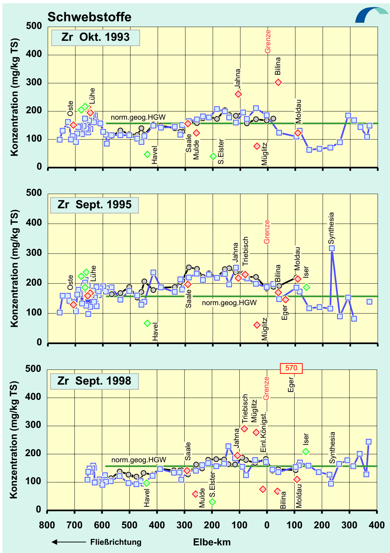
Abb.39c: Vergleich der Zirkonium -Konzentrationen in der Schwebstoff -Trockensubstanz (TS) der Elbe von der Mündung bis zur Quelle: Oktober 1993 / Sept. 1995 / Sept. 1998
