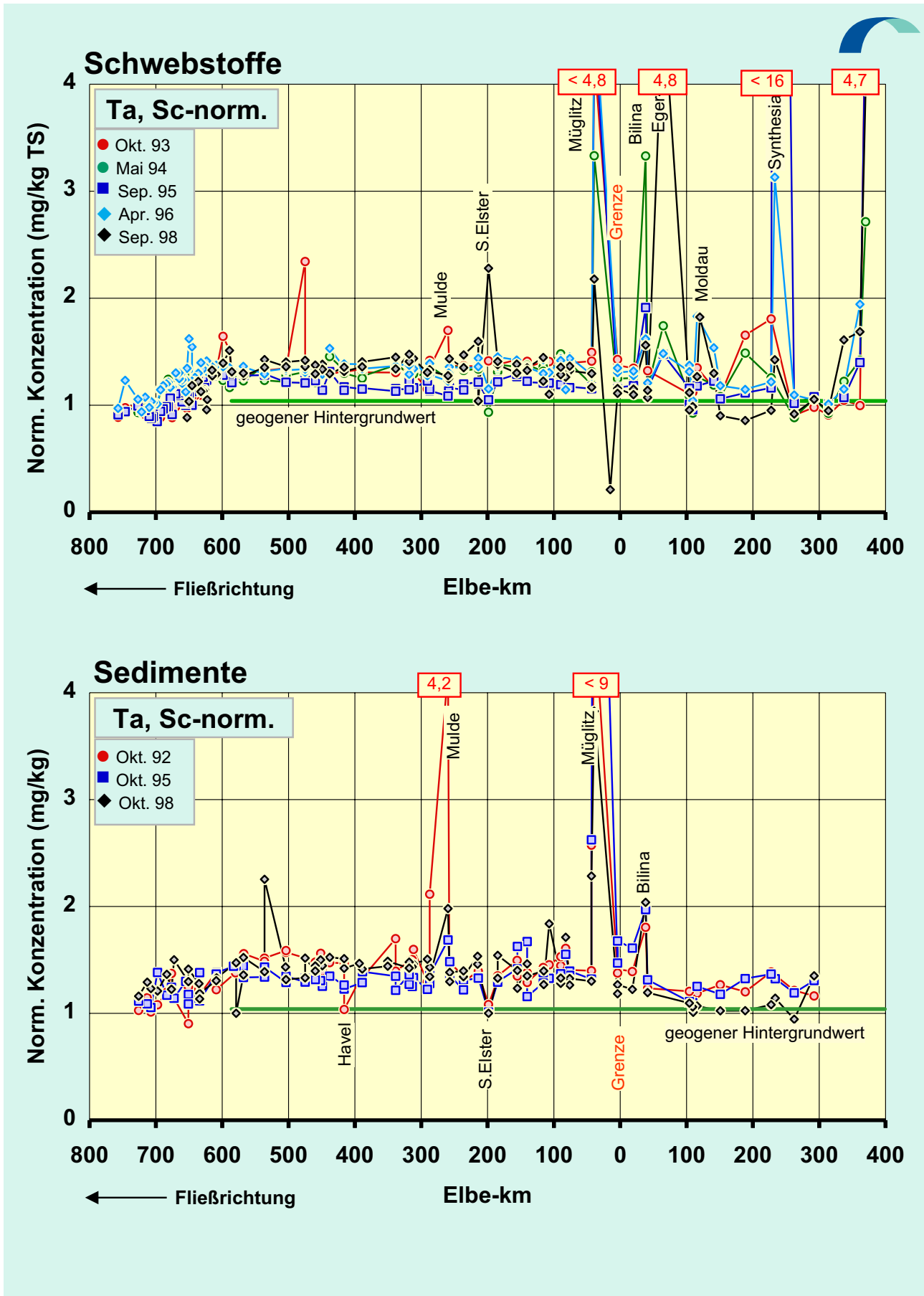
Abb.63f: Vergleich der Sc-normierten Tantal -Konzentrationen in der Schwebstoff -Trocken- substanz (TS) (oben) und der < 20-µm-Fraktion der Sedimente (unten) der Elbe von der Mündung bis zur Quelle für diverse Probenahmezeitpunkte. Normierung : C_{Ta}^{norm} = C_{Ta} / C_{Sc} \cdot C_{Sc}^0 , mit C_{Sc}^0 = 13 \text{ mg/kg}
