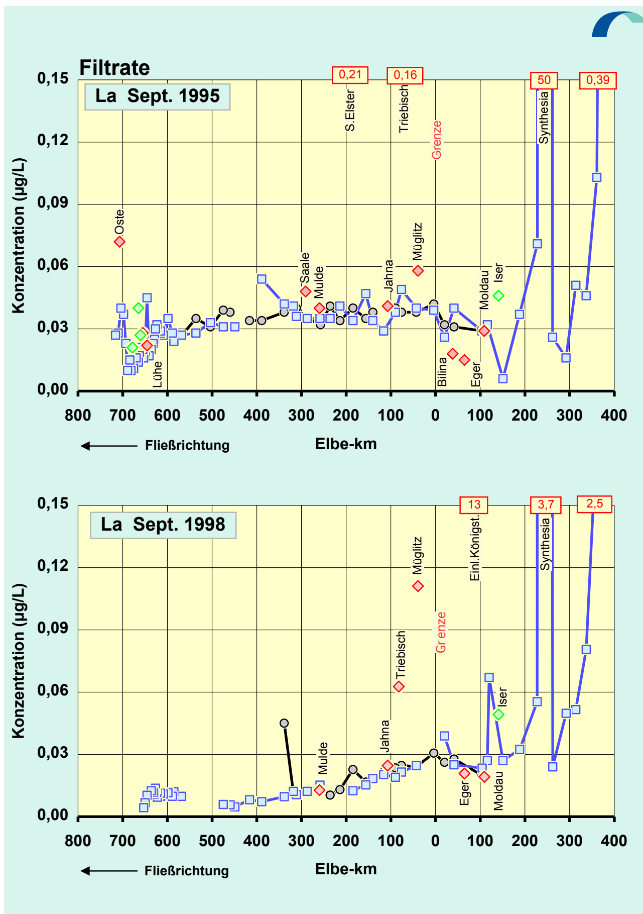
Abb.48a: Vergleich der Lanthan -Konzentrationen in den Filtraten der Elbe von der Mündung bis zur Quelle: September 1995 / September 1998 / (Oktober 1993 keine Messwerte)
