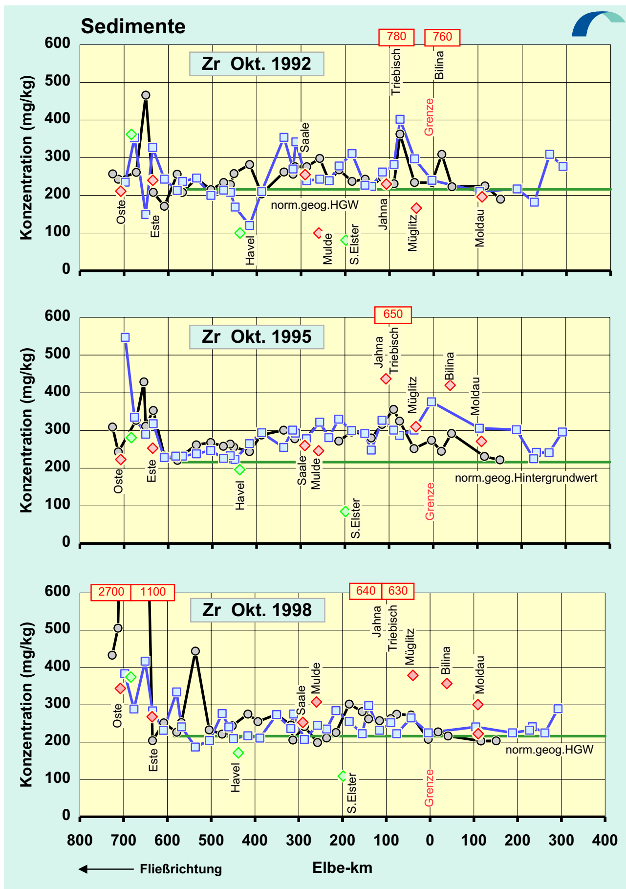
Abb.39e: Vergleich der Zirkonium -Konzentrationen der Elbe- Sedimente (<20µm-Fraktion) von der Mündung bis zur Quelle: Oktober 1992 / Oktober 1995 / Oktober 1998
