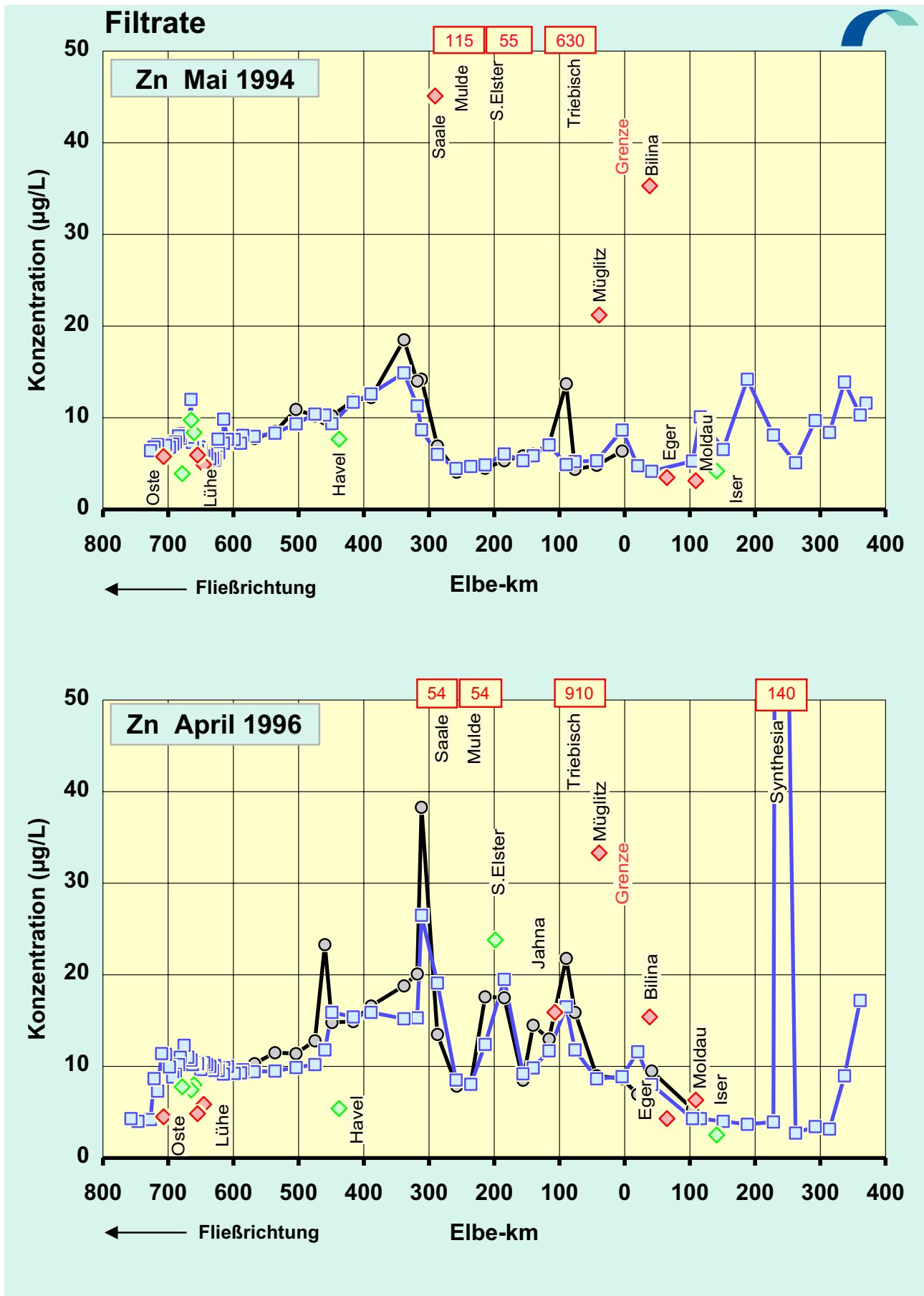
Abb.30b: Vergleich der Zink -Konzentrationen in den Filtraten der Elbe von der Mündung bis zur Quelle: Mai 1994 / April 1996
