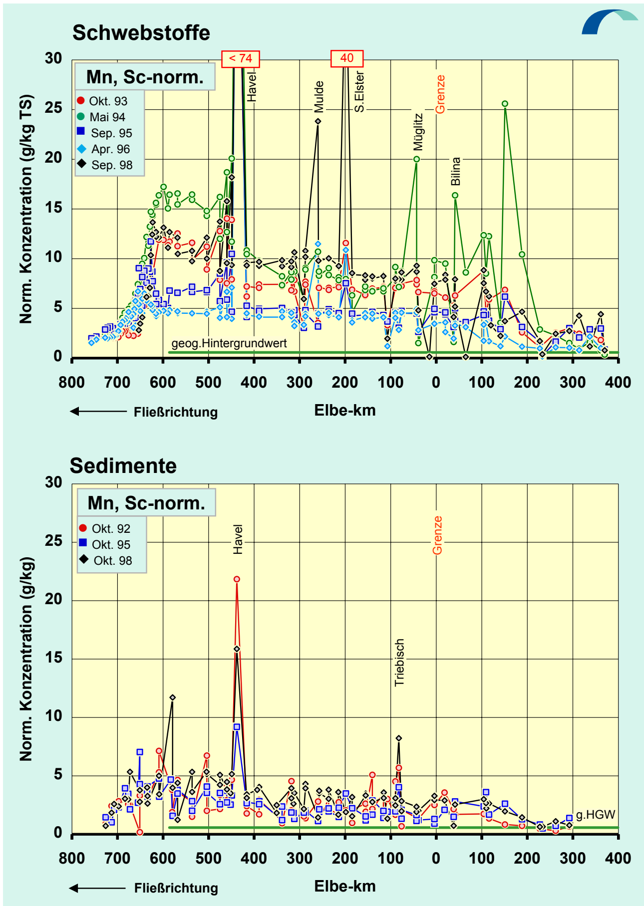
Abb.25f: Vergleich der Sc-normierten Mangan -Konzentrationen in der Schwebstoff -Trocken- substanz (TS) (oben) und der < 20-µm-Fraktion der Sedimente (unten) der Elbe von der Mündung bis zur Quelle für diverse Probennahmezeitpunkte. Normierung : C_{Mn}^{norm} = C_{Mn} / C_{Sc} \cdot C_{Sc}^0 , mit C_{Sc}^0 = 13 \text{ mg/kg}
