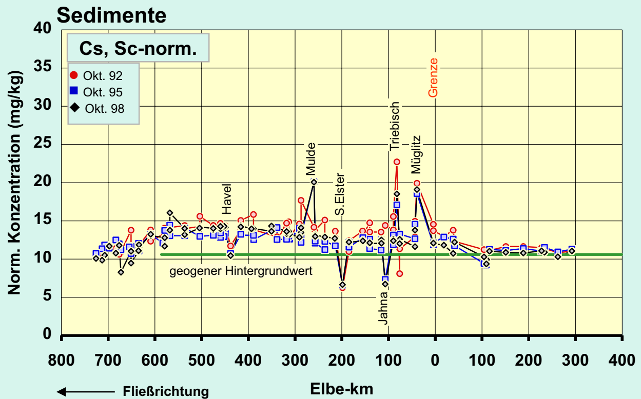
Abb.46f: Vergleich der Sc-normierten Cäsium -Konzentrationen in der Schwebstoff -Trocken-substanz (TS) (oben) und der < 20-µm-Fraktion der Sedimente (unten) der Elbe von der Mündung bis zur Quelle für diverse Probenahmezeitpunkte. Normierung : C_{Cs}^{norm} = C_{Cs} / C_{Sc} \cdot C_{Sc}^0 , mit C_{Sc}^0 = 13 \text{ mg/kg}
