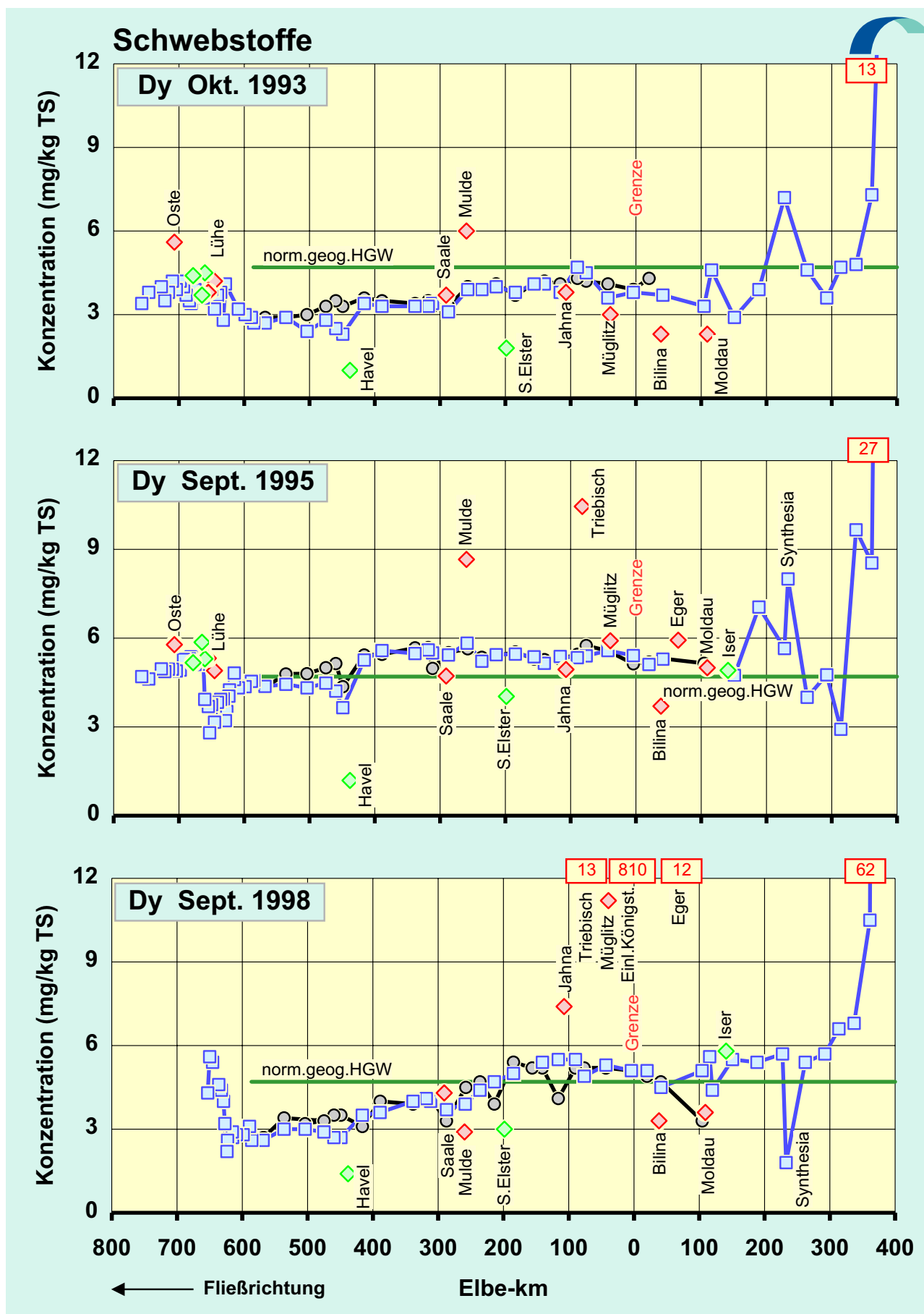
Abb.56c: Vergleich der Dysprosium -Konzentrationen in der Schwebstoff -Trockensubstanz(TS) der Elbe von der Mündung bis zur Quelle: Oktober 1993 / Sept. 1995 / Sept. 1998 Legende: ■ rechtes Ufer und Flussmitte ● linkes Ufer ◆ Nebenfluss links ◆ Nebenfluss rechts
