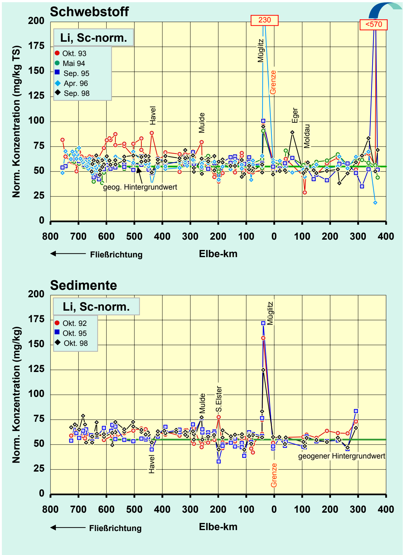
Abb.11f: Vergleich der Sc-normierten Lithium -Konzentrationen in der Schwebstoff -Trocken- substanz (TS) (oben) und der < 20-µm-Fraktion der Sedimente (unten) der Elbe von der Mündung bis zur Quelle für diverse Probenahmezeitpunkte. Normierung : C_{Li}^{norm} = C_{Li} / C_{Sc} \cdot C_{Sc}^0 , mit C_{Sc}^0 = 13 \text{ mg/kg}
