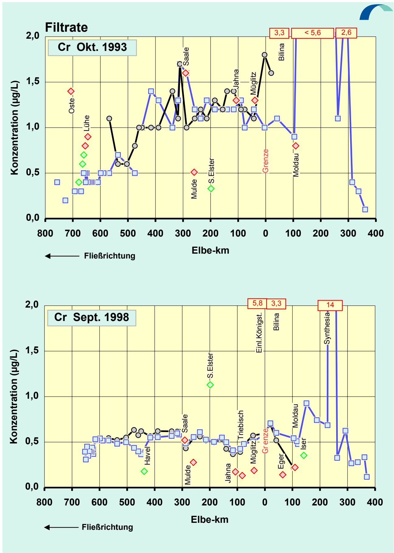
Abb.24a: Vergleich der Chrom -Konzentrationen in den Filtraten der Elbe von der Mündung bis zur Quelle: Oktober 1993 / September 1998 / (September 1995 keine Messwerte)
