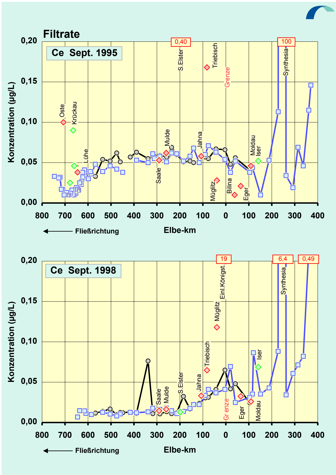
Abb.49a: Vergleich der Ce -Konzentrationen in den Filtraten der Elbe von der Mündung bis zur Quelle: September 1995 / September 1998 / (Oktober 1993 keine Messwerte)
