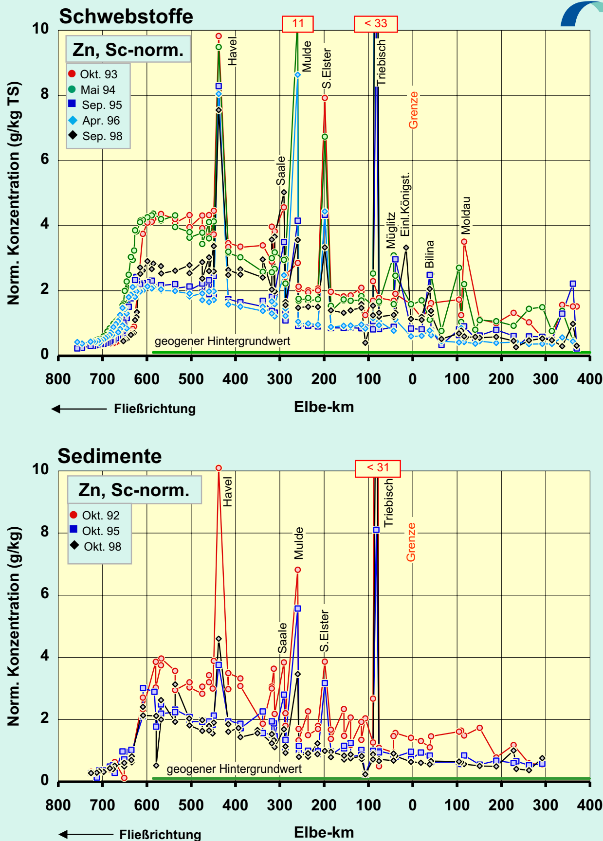
Abb.30f: Vergleich der Sc-normierten Zink -Konzentrationen in der Schwebstoff -Trocken- substanz (TS) (oben) und der < 20-µm-Fraktion der Sedimente (unten) der Elbe von der Mündung bis zur Quelle für diverse Probenahmezeitpunkte. Normierung : C_{Zn}^{norm} = C_{Zn} / C_{Sc} \cdot C_{Sc}^0 , mit C_{Sc}^0 = 13 \text{ mg/kg}
