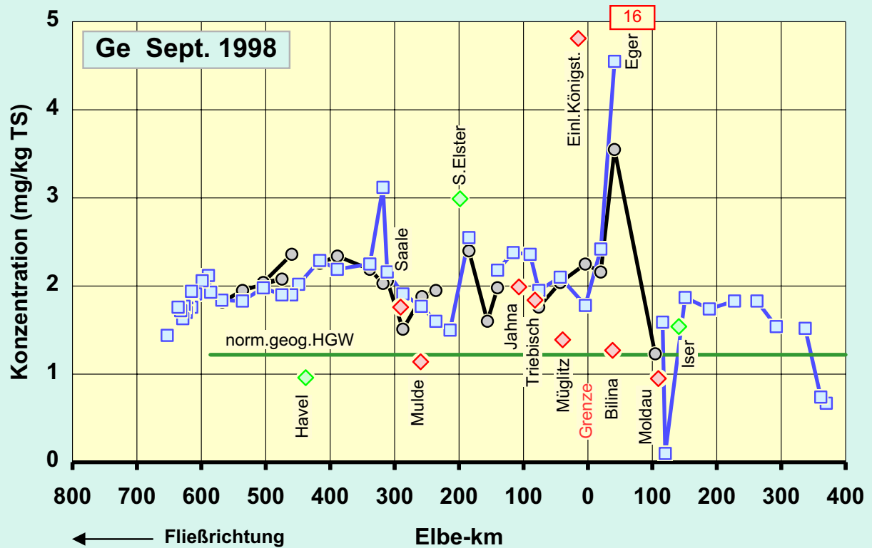
Abb.32c: Vergleich der Germanium -Konzentrationen in der Schwebstoff -Trockensubstanz (TS) der Elbe von der Mündung bis zur Quelle: Sept. 1995 / Sept. 1998 / (Okt. 1993 keine Messwerte)
