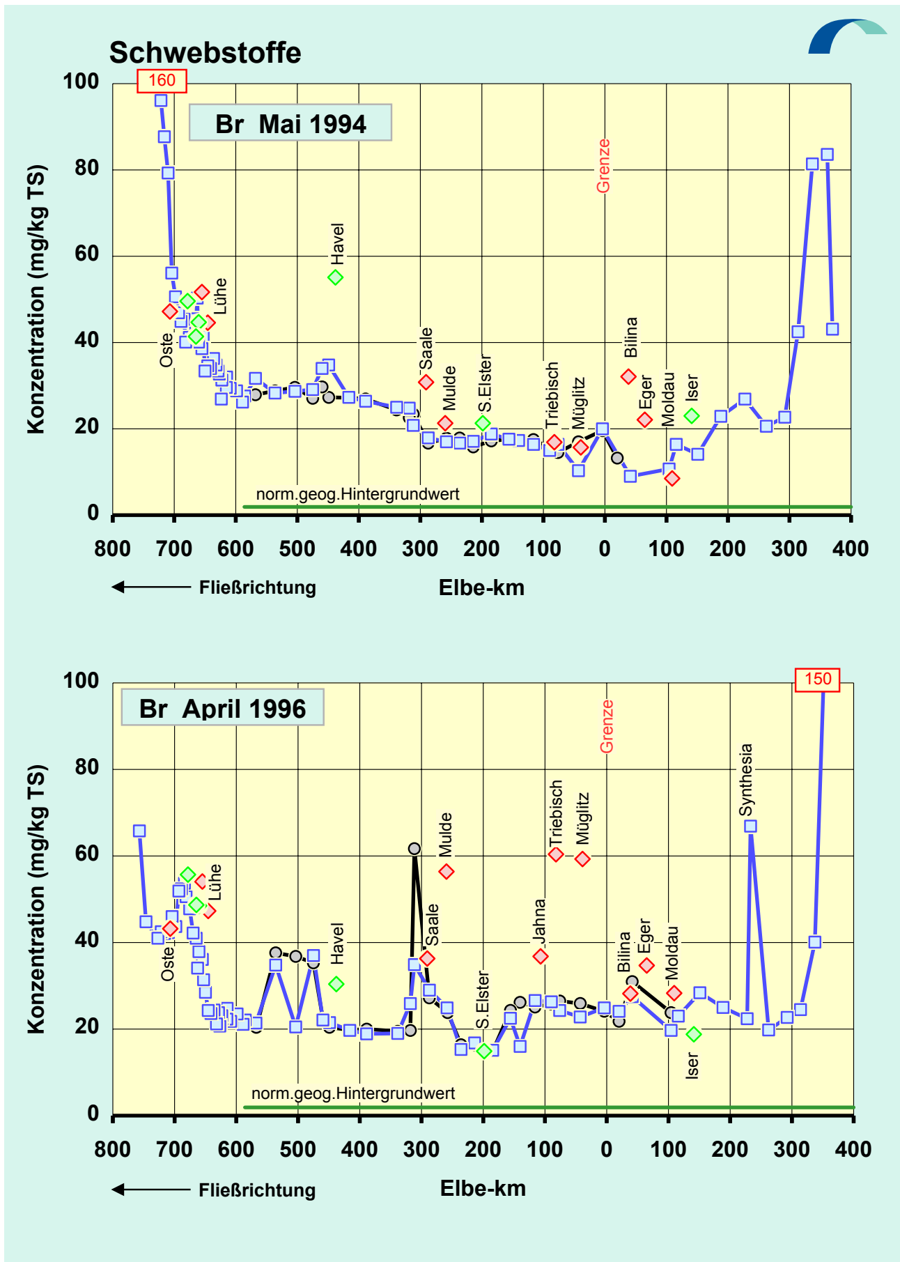
Abb.35d: Vergleich der Brom -Konzentrationen in der Schwebstoff -Trockensubstanz (TS) der Elbe von der Mündung bis zur Quelle: Mai 1994 / April 1996
