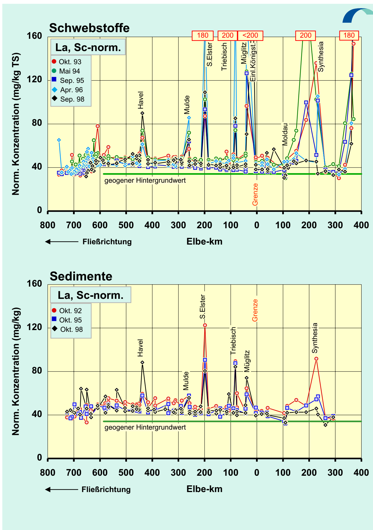
Abb.48f: Vergleich der Sc-normierten Lanthan -Konzentrationen in der Schwebstoff -Trocken- substanz (TS) (oben) und der < 20-µm-Fraktion der Sedimente (unten) der Elbe von der Mündung bis zur Quelle für diverse Probenahmezeitpunkte. Normierung : C_{La}^{norm} = C_{La} / C_{Sc} \cdot C^0_{Sc} , mit C^0_{Sc} = 13 \text{ mg/kg}
