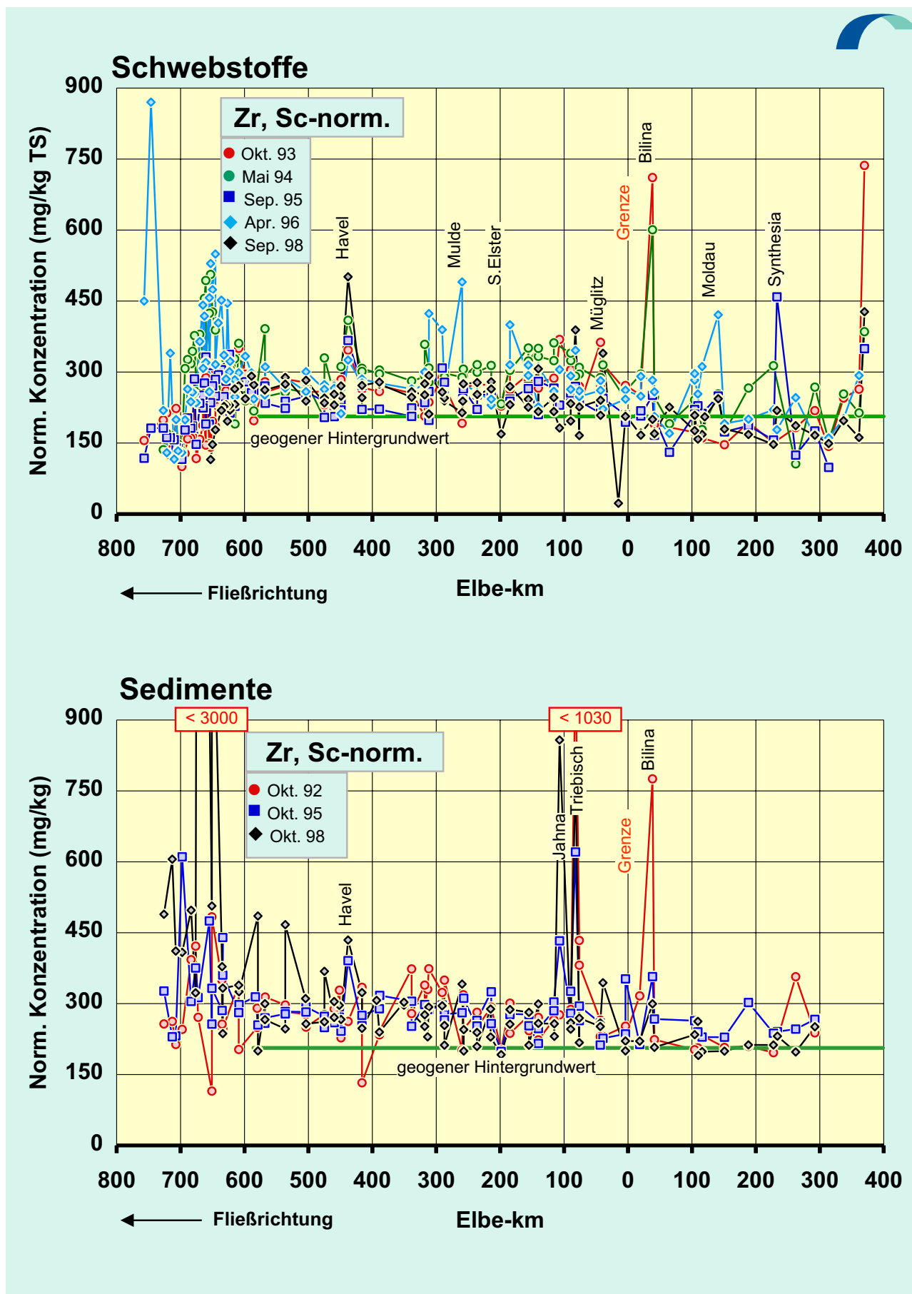
Abb.39f: Vergleich der Sc-normierten Zirkonium -Konzentrationen in der Schwebstoff -Trocken- substanz (TS) (oben) und der < 20-µm-Fraktion der Sedimente (unten) der Elbe von der Mündung bis zur Quelle für diverse Probennahmezeitpunkte. Normierung : C_{Zr}^{norm} = C_{Zr} / C_{Sc} \cdot C_{Sc}^0 , mit C_{Sc}^0 = 13 \text{ mg/kg}
