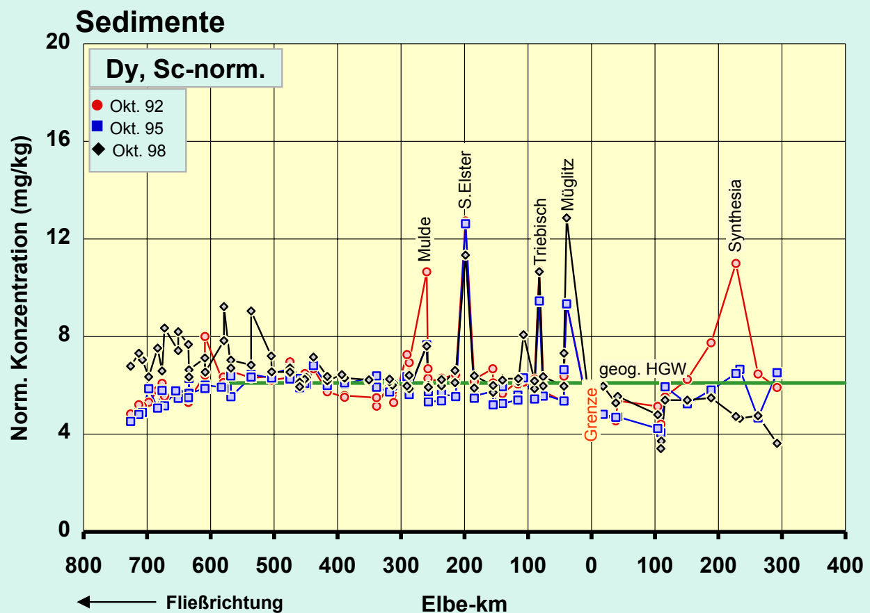
Abb.56f: Vergleich der Sc-normierten Dysprosium -Konzentrationen in der Schwebstoff -Trokensubstanz (TS) (oben) und der < 20-µm-Fraktion der Sedimente (unten) der Elbe von der Mündung bis zur Quelle für diverse Probennahmezeitpunkte. Normierung : C_{Dy}^{norm} = C_{Dy} / C_{Sc} \cdot C_{Sc}^0 , mit C_{Sc}^0 = 13 \text{ mg/kg}
