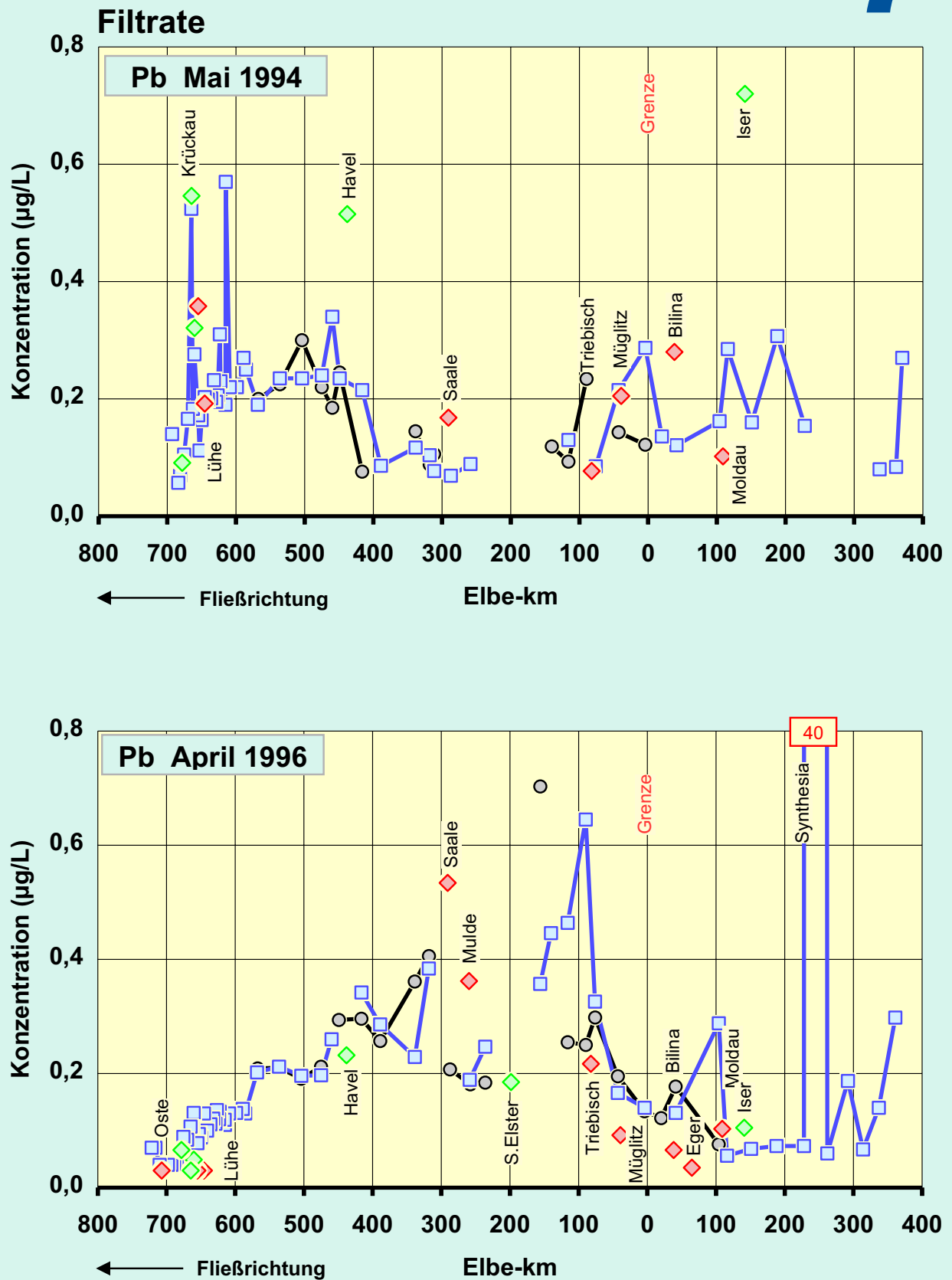
Abb.68b: Vergleich der Blei -Konzentrationen in den Filtraten der Elbe von der Mündung bis zur Quelle: Mai 1994 / April 1996
