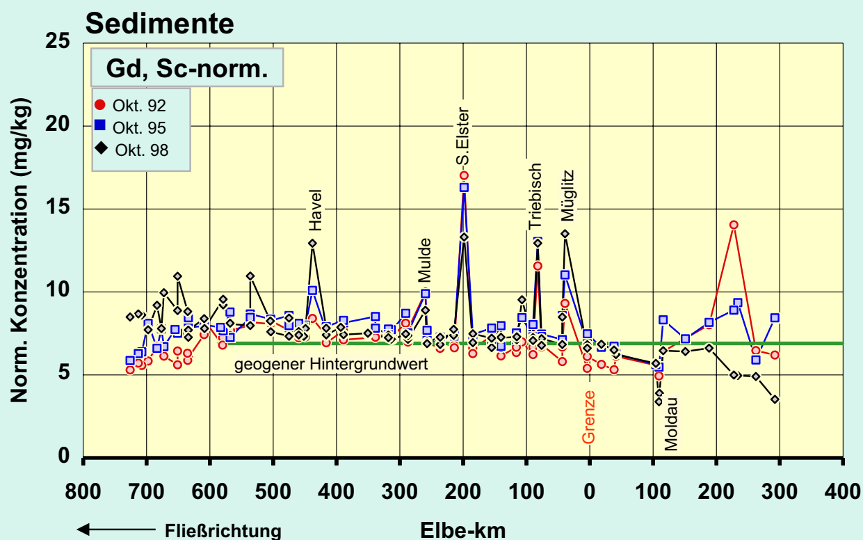
Abb.54f: Vergleich der Sc-normierten Gadolinium -Konzentrationen in der Schwebstoff -Trokensubstanz (TS) (oben) und der < 20-µm-Fraktion der Sedimente (unten) der Elbe von der Mündung bis zur Quelle für diverse Probenahmezeitpunkte. Normierung : C_{Gd}^{norm} = C_{Gd} / C_{Sc} \cdot C_{Sc}^0 , mit C_{Sc}^0 = 13 \text{ mg/kg}
