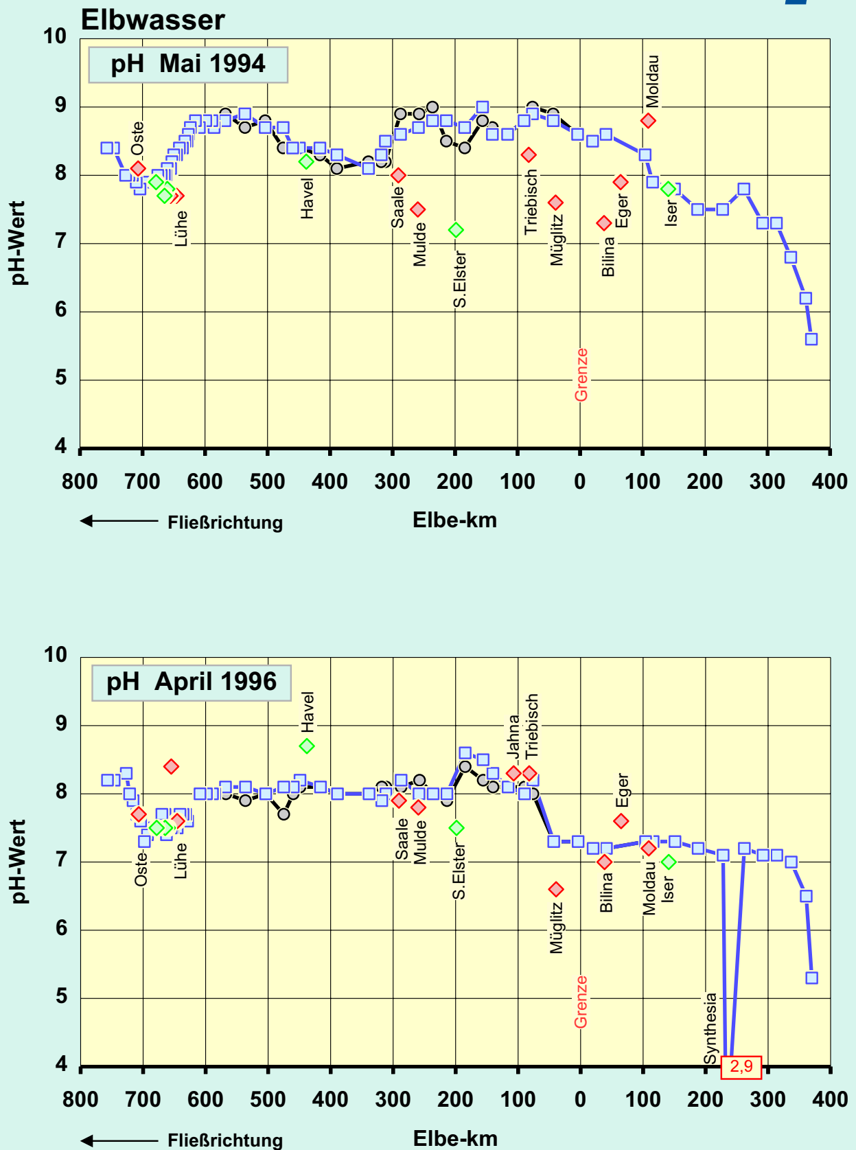
Abb.4b: Vergleich der pH-Werte in der Elbe von der Mündung bis zur Quelle: Mai 1994 / April 1996
