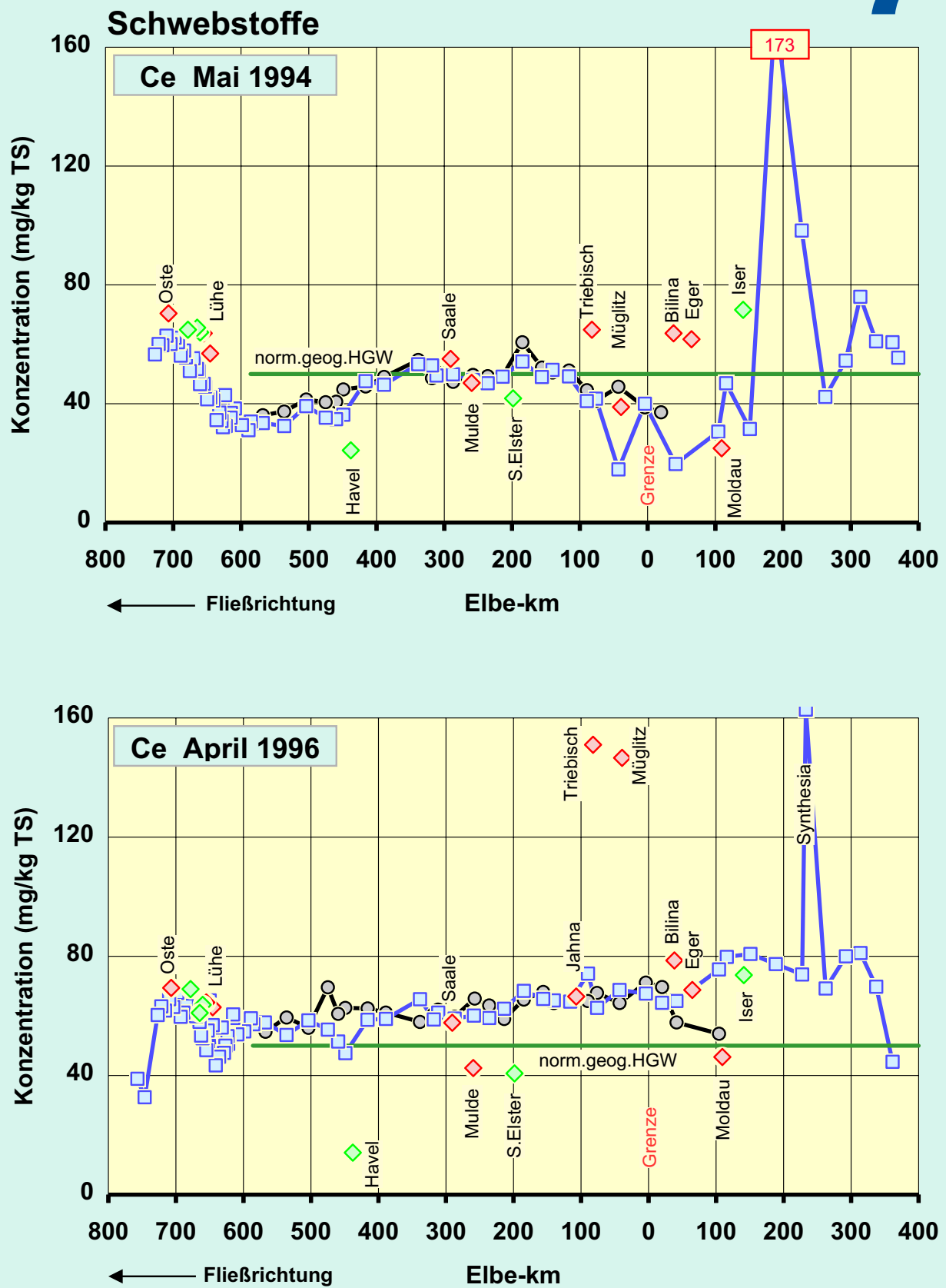
Abb.49d: Vergleich der Ce -Konzentrationen in der Schwebstoff -Trockensubstanz (TS) der Elbe von der Mündung bis zur Quelle: Mai 1994 / April 1996
