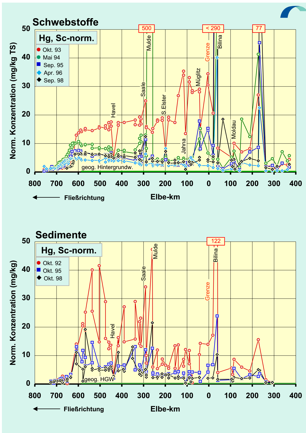
Abb.66f: Vergleich der Sc-normierten Quecksilber -Konzentrationen in der Schwebstoff -Trockensubstanz (TS) (oben) und der < 20-µm-Fraktion der Sedimente (unten) der Elbe von der Mündung bis zur Quelle für diverse Probenahmezeitpunkte. Normierung : C_{Hg}^{norm} = C_{Hg} / C_{Sc} \cdot C_{Sc}^0 , mit C_{Sc}^0 = 13 \text{ mg/kg}
