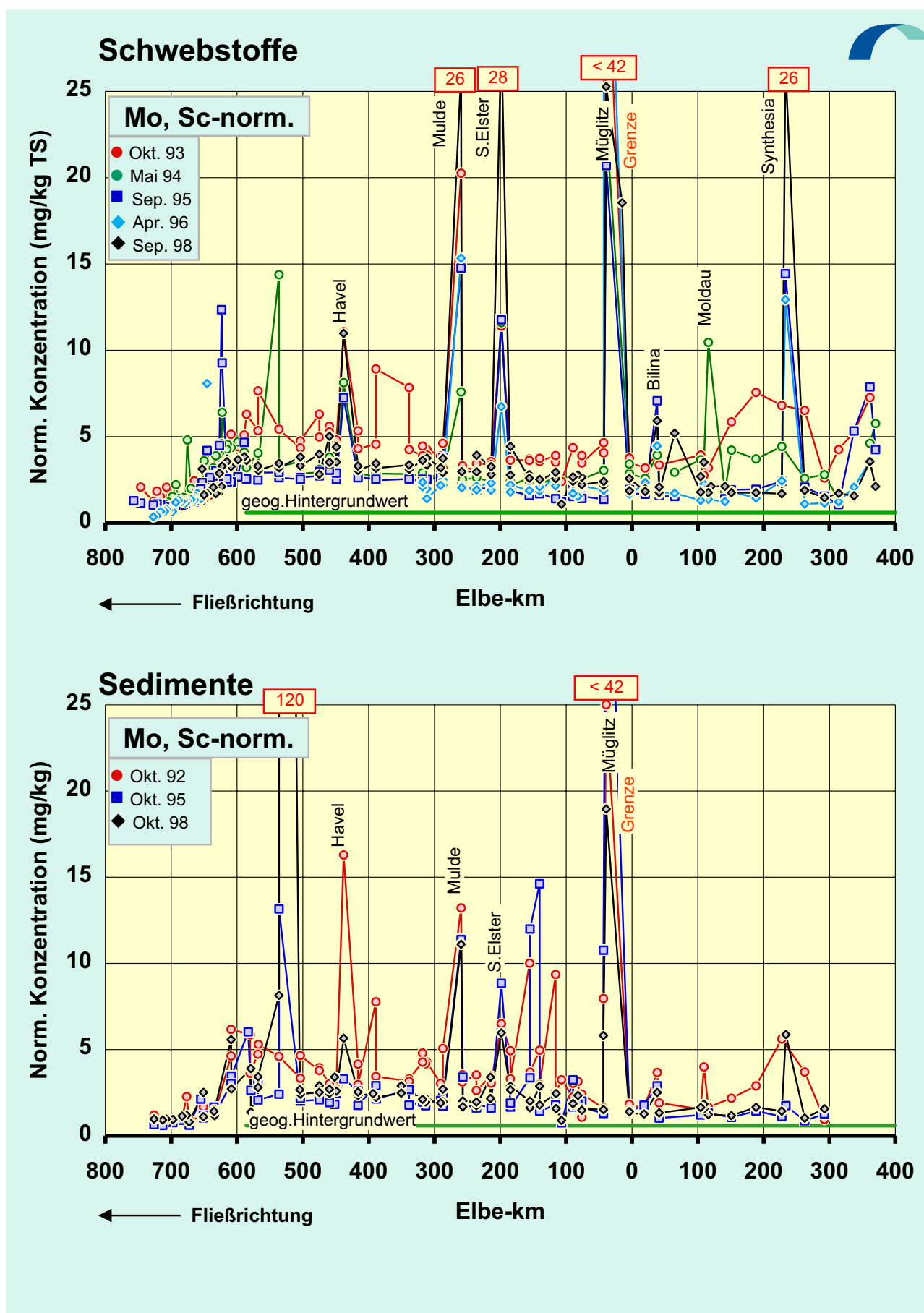
Abb.41f: Vergleich der Sc-normierten Molybdän -Konzentrationen in der Schwebstoff -Trocken- substanz (TS) (oben) und der < 20-µm-Fraktion der Sedimente (unten) der Elbe von der Mündung bis zur Quelle für diverse Probenahmezeitpunkte. Normierung : C_{Mo}^{norm} = C_{Mo} / C_{Sc} \cdot C_{Sc}^0 , mit C_{Sc}^0 = 13 \text{ mg/kg}
