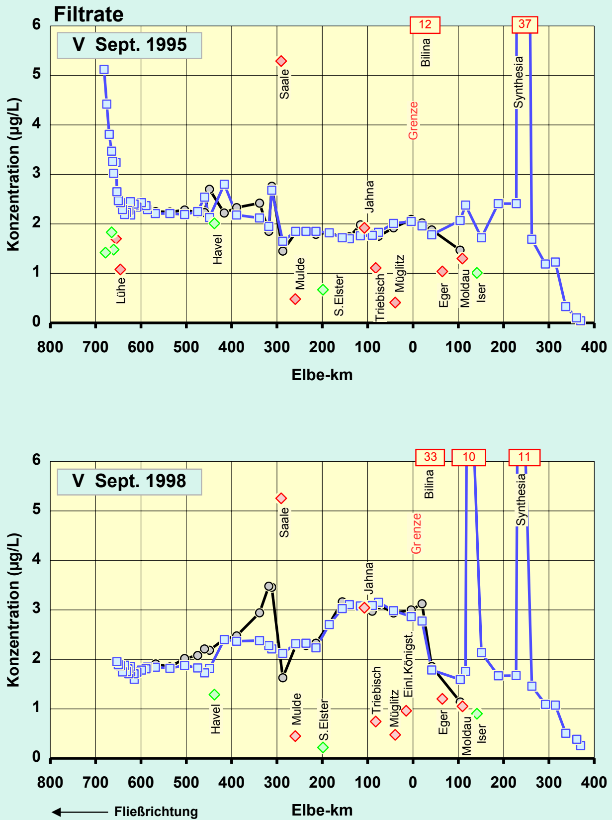
Abb.23a: Vergleich der Vanadium -Konzentrationen in den Filtraten der Elbe von der Mündung bis zur Quelle: September 1995 / September 1998 / (Oktober 1993 keine Messwerte) Legende: ■ rechtes Ufer und Flussmitte ● linkes Ufer ◆ Nebenfluss links ◆ Nebenfluss rechts
