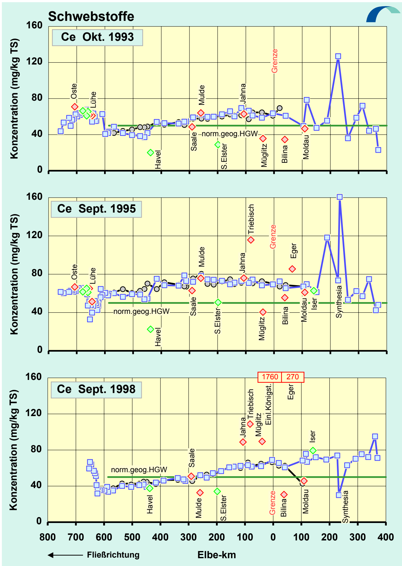
Abb.49c: Vergleich der Cer -Konzentrationen in der Schwebstoff -Trockensubstanz (TS) der Elbe von der Mündung bis zur Quelle: Oktober 1993 / Sept. 1995 / Sept. 1998
