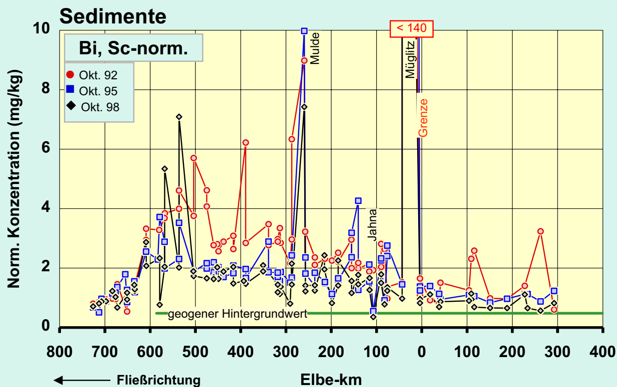
Abb.69f: Vergleich der Sc-normierten Bismut -Konzentrationen in der Schwebstoff -Trocken- substanz (TS) (oben) und der < 20-µm-Fraktion der Sedimente (unten) der Elbe von der Mündung bis zur Quelle für diverse Probenahmezeitpunkte. Normierung : C_{Bi}^{norm} = C_{Bi} / C_{Sc} \cdot C^0_{Sc} , mit C^0_{Sc} = 13 \text{ mg/kg}
