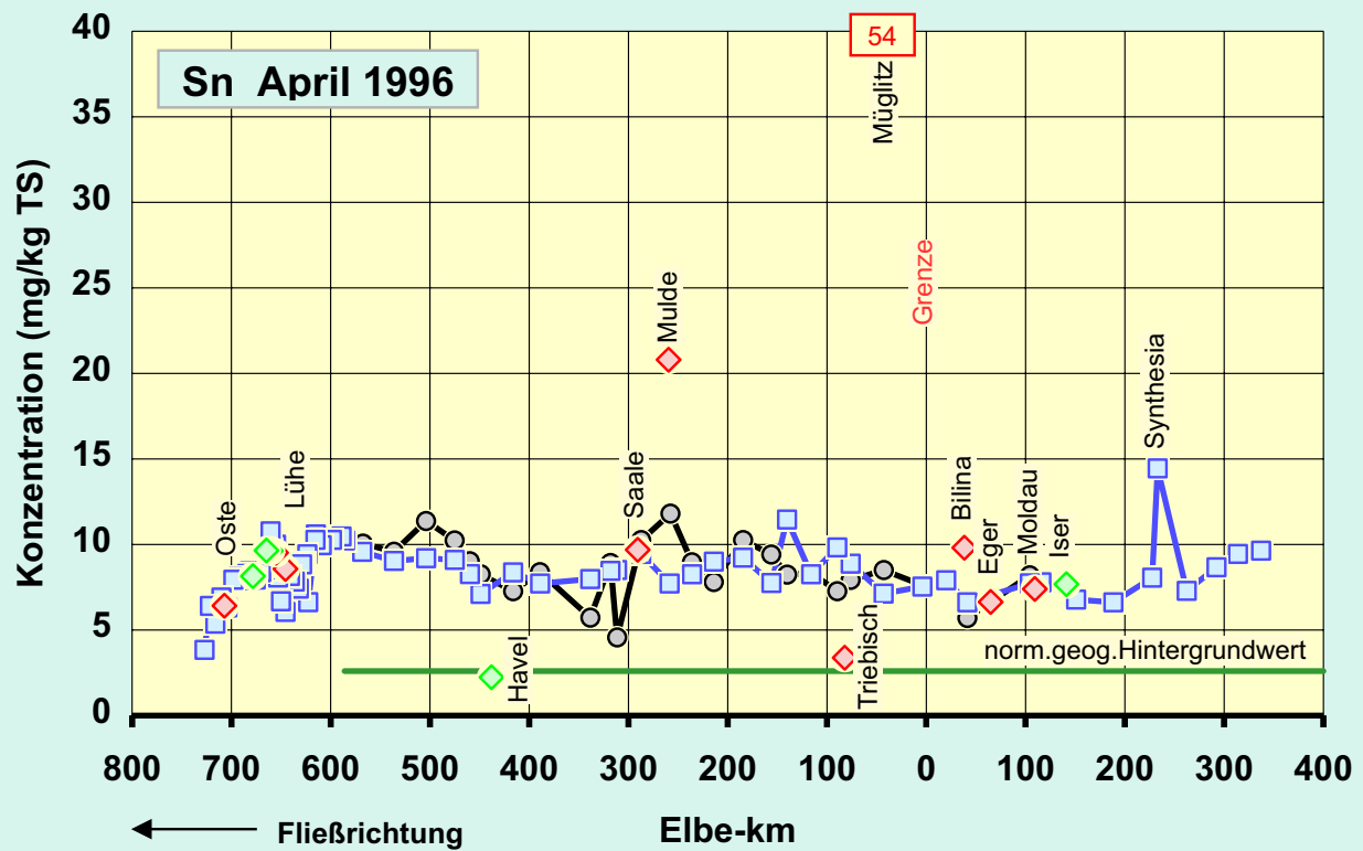
Abb.44d: Vergleich der Zinn -Konzentrationen in der Schwebstoff -Trockensubstanz (TS) der Elbe von der Mündung bis zur Quelle: Mai 1994 / April 1996
