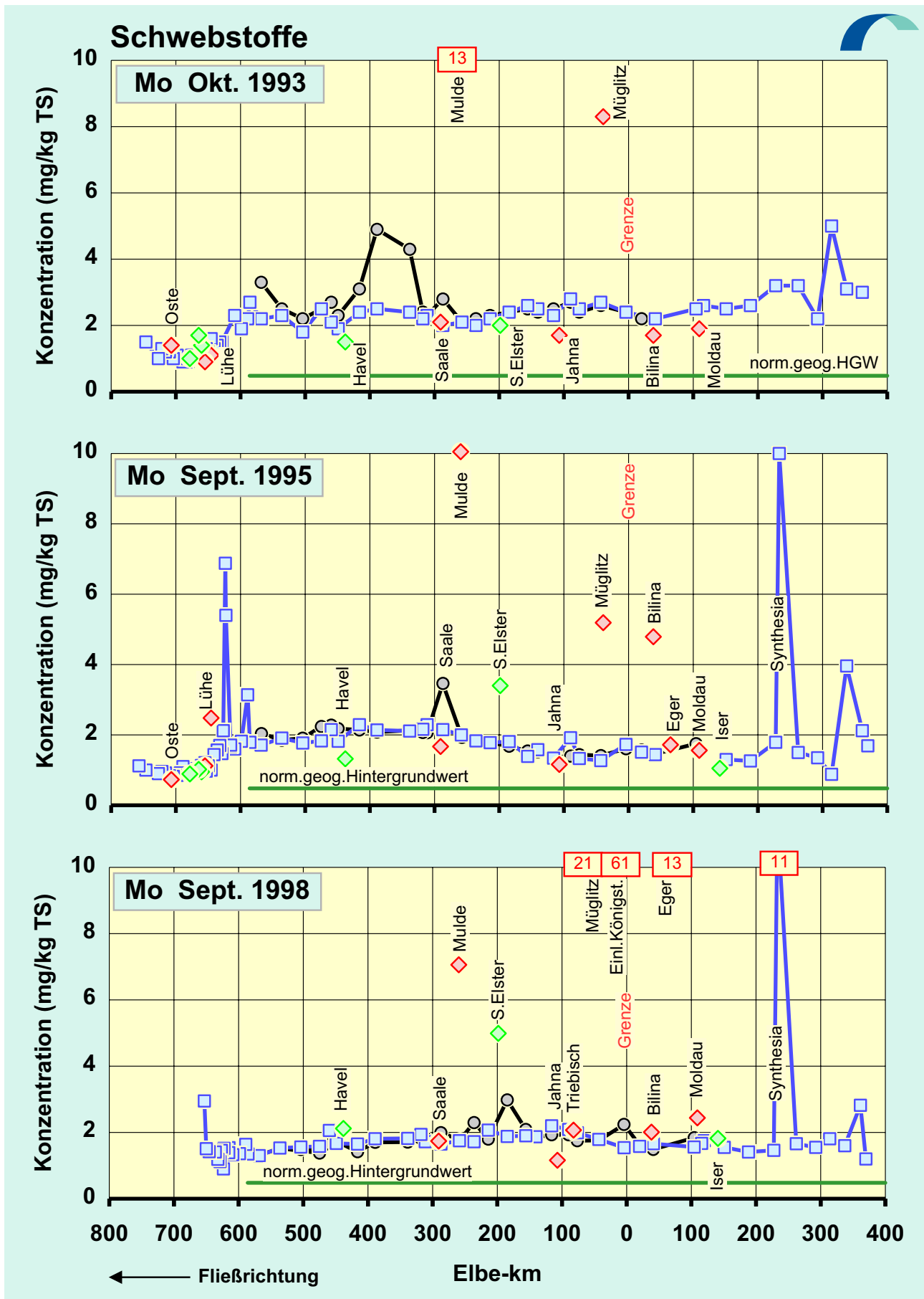
Abb.41c: Vergleich der Molybdän -Konzentrationen in der Schwebstoff -Trockensubstanz (TS) der Elbe von der Mündung bis zur Quelle: Oktober 1993 / Sept. 1995 / Sept. 1998
