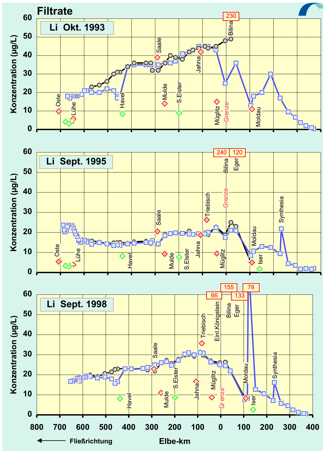
Abb.11a: Vergleich der Lithium -Konzentrationen in den Filtraten der Elbe von der Mündung bis zur Quelle: Oktober 1993 / September 1995 / September 1998
