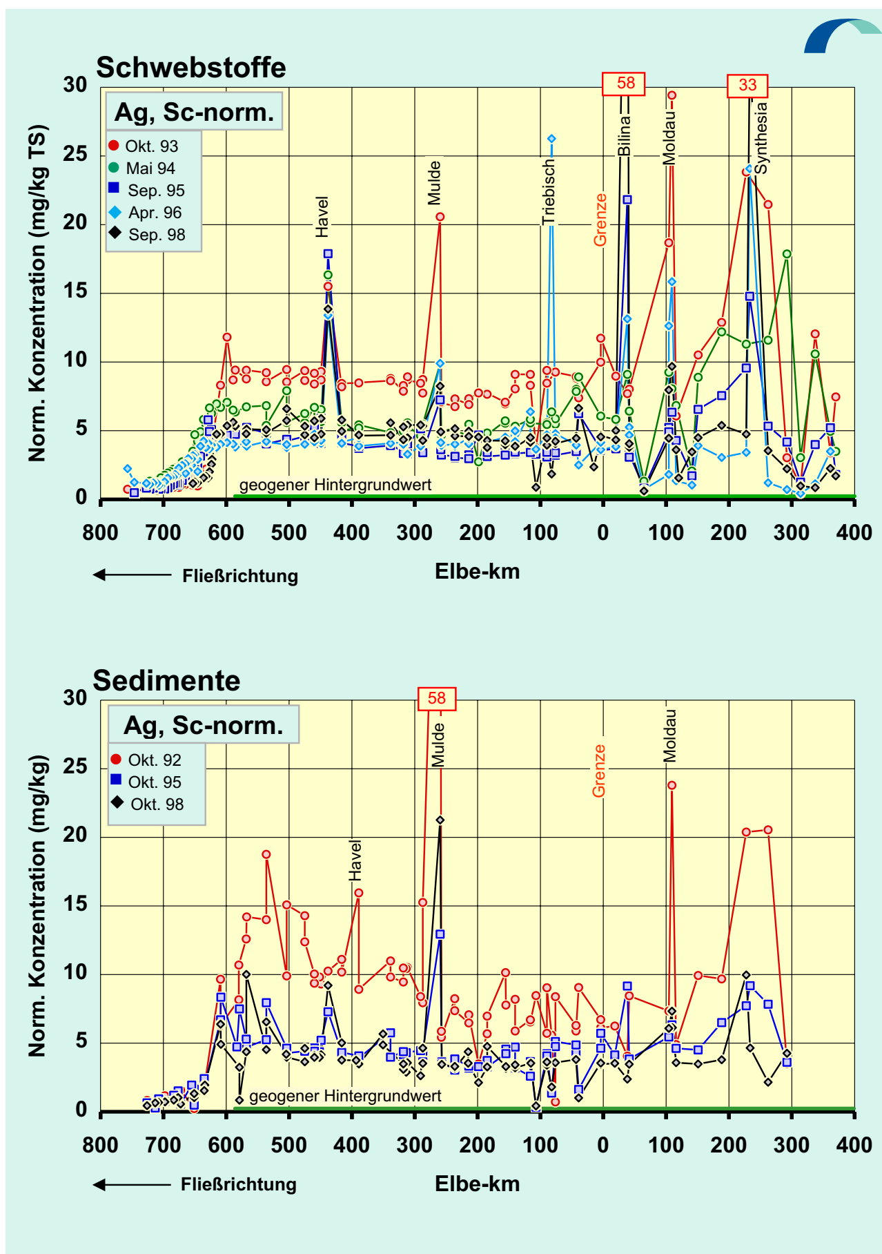
Abb.42f: Vergleich der Sc-normierten Silber -Konzentrationen in der Schwebstoff -Trocken- substanz (TS) (oben) und der < 20-µm-Fraktion der Sedimente (unten) der Elbe von der Mündung bis zur Quelle für diverse Probenahmezeitpunkte. Normierung : C_{Ag}^{norm} = C_{Ag} / C_{Sc} \cdot C_{Sc}^0 , mit C_{Sc}^0 = 13 \text{ mg/kg}
