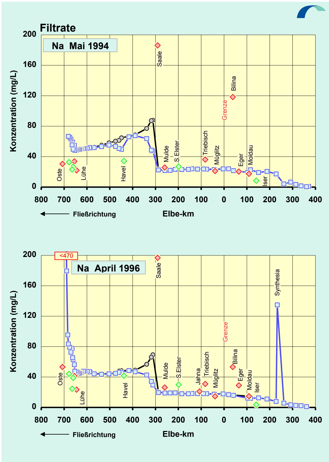
Abb.14b: Vergleich der Natrium -Konzentrationen in den Filtraten der Elbe von der Mündung bis zur Quelle: Mai 1994 / April 1996
