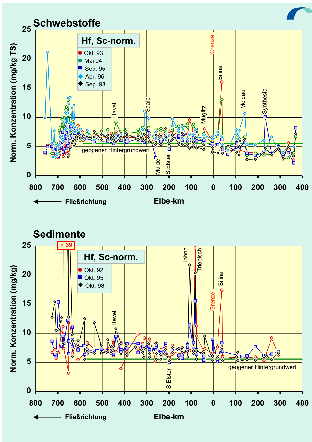
Abb.62f: Vergleich der Sc-normierten Hafnium -Konzentrationen in der Schwebstoff -Trocken- substanz (TS) (oben) und der < 20-µm-Fraktion der Sedimente (unten) der Elbe von der Mündung bis zur Quelle für diverse Probenahmezeitpunkte. Normierung : C_{Hf}^{norm} = C_{Hf} / C_{Sc} \cdot C_{Sc}^0 , mit C_{Sc}^0 = 13 \text{ mg/kg}
