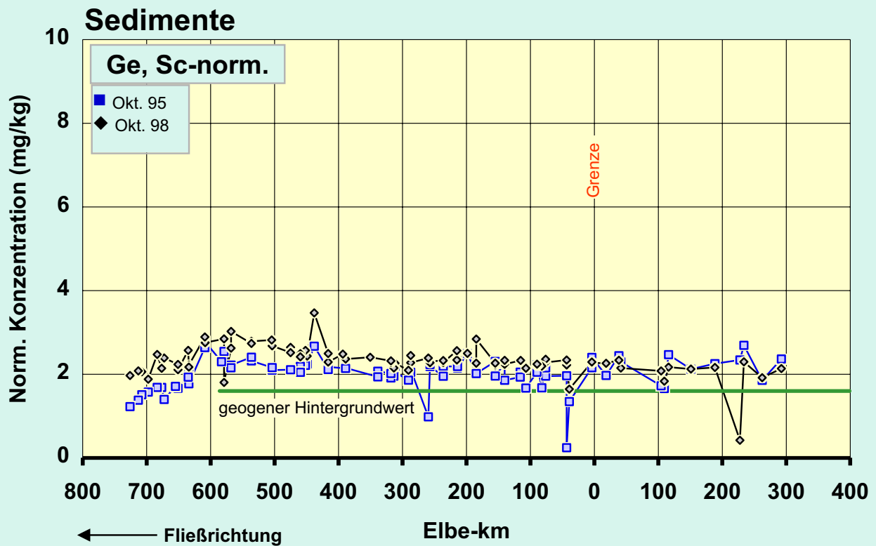
Abb.32f: Vergleich der Sc-normierten Germanium -Konzentrationen in der Schwebstoff -Trokensubstanz (TS) (oben) und der < 20-µm-Fraktion der Sedimente (unten) der Elbe von der Mündung bis zur Quelle für diverse Probenahmezeitpunkte. Normierung : C_{Ge}^{norm} = C_{Ge} / C_{Sc} \cdot C_{Sc}^0 , mit C_{Sc}^0 = 13 \text{ mg/kg}
