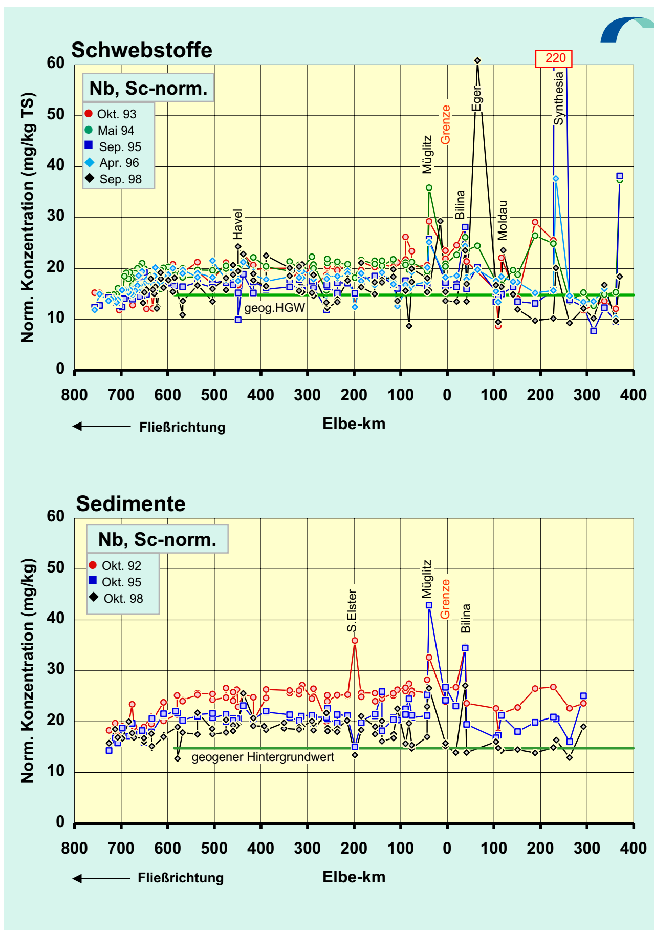
Abb.40f: Vergleich der Sc-normierten Niob -Konzentrationen in der Schwebstoff -Trocken- substanz (TS) (oben) und der < 20-µm-Fraktion der Sedimente (unten) der Elbe von der Mündung bis zur Quelle für diverse Probenahmezeitpunkte. Normierung : C_{Nb}^{norm} = C_{Nb} / C_{Sc} \cdot C_{Sc}^0 , mit C_{Sc}^0 = 13 \text{ mg/kg}
