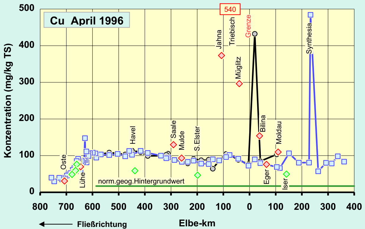
Abb.29d: Vergleich der Kupfer -Konzentrationen in der Schwebstoff -Trockensubstanz (TS) der Elbe von der Mündung bis zur Quelle: Mai 1994 / April 1996
