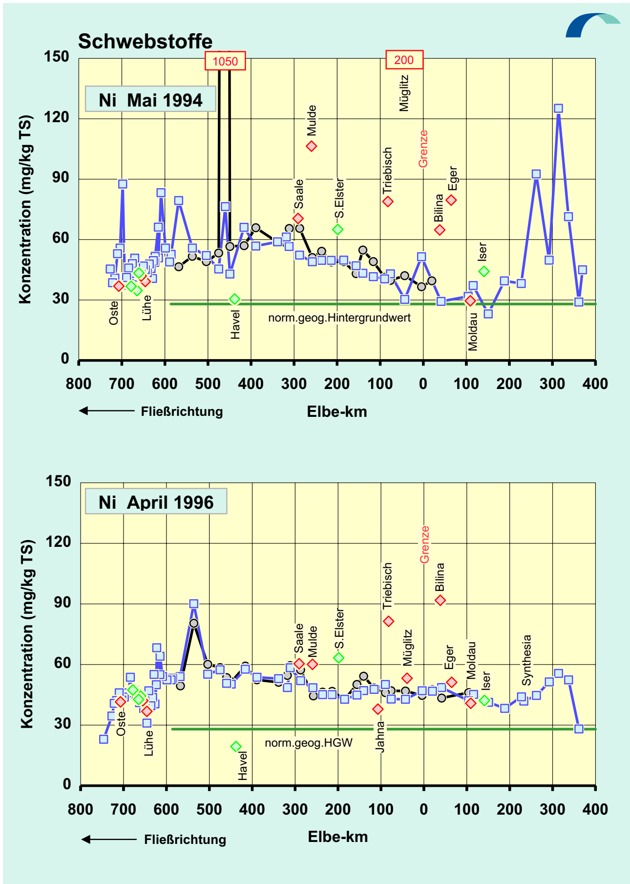
Abb.28d: Vergleich der Nickel -Konzentrationen in der Schwebstoff -Trockensubstanz (TS) der Elbe von der Mündung bis zur Quelle: Mai 1994 / April 1996 Legende: ■ rechtes Ufer und Flussmitte ● linkes Ufer ◆ Nebenfluss links ◆ Nebenfluss rechts
