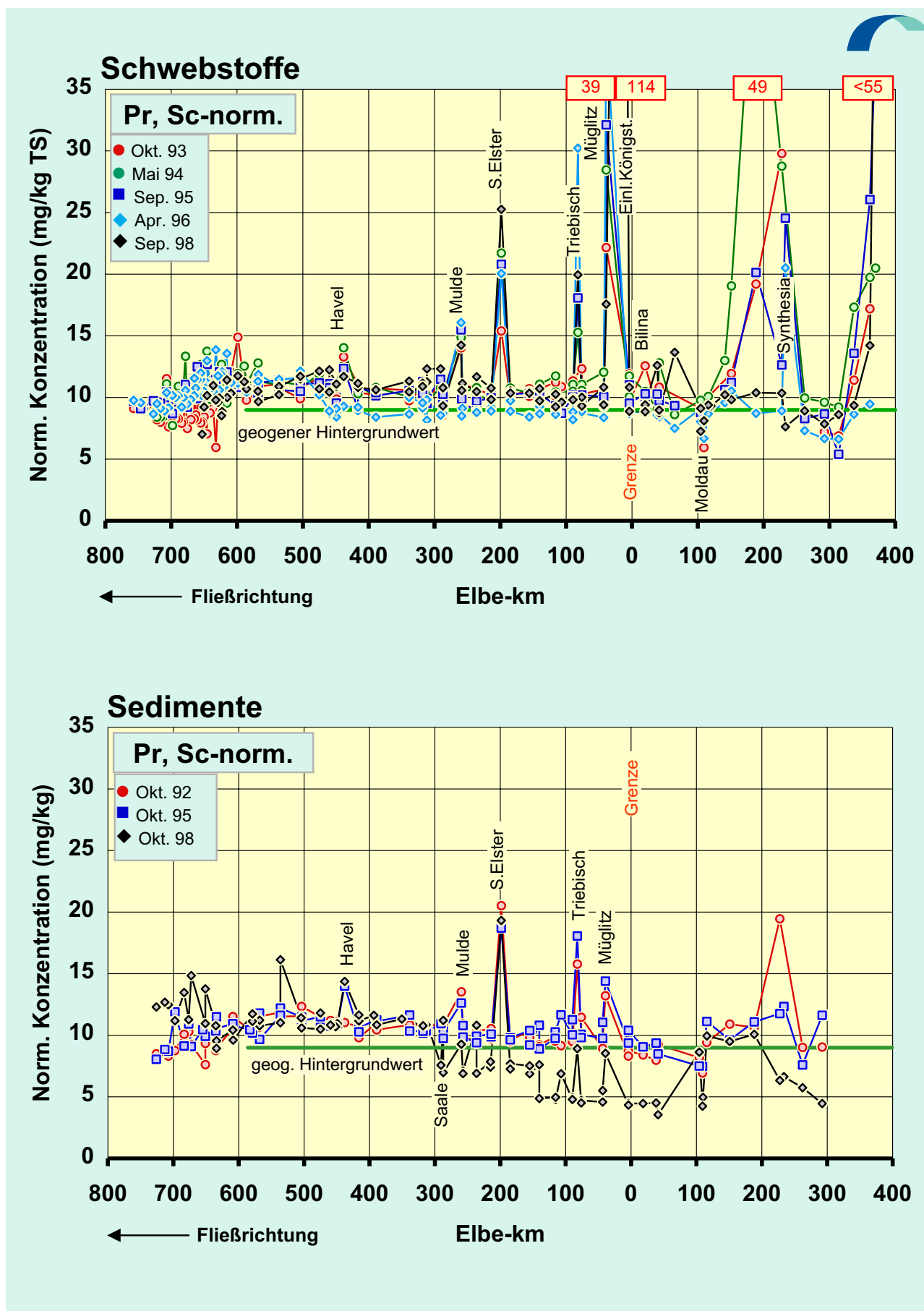
Abb.50f: Vergleich der Sc-normierten Praseodym -Konzentrationen in der Schwabstoff -Trokensubstanz (TS) (oben) und der < 20-µm-Fraktion der Sedimente (unten) der Elbe von der Mündung bis zur Quelle für diverse Probenahmezeitpunkte. Normierung : C_{Pr}^{norm} = C_{Pr} / C_{Sc} \cdot C^0_{Sc} , mit C^0_{Sc} = 13 \text{ mg/kg}
