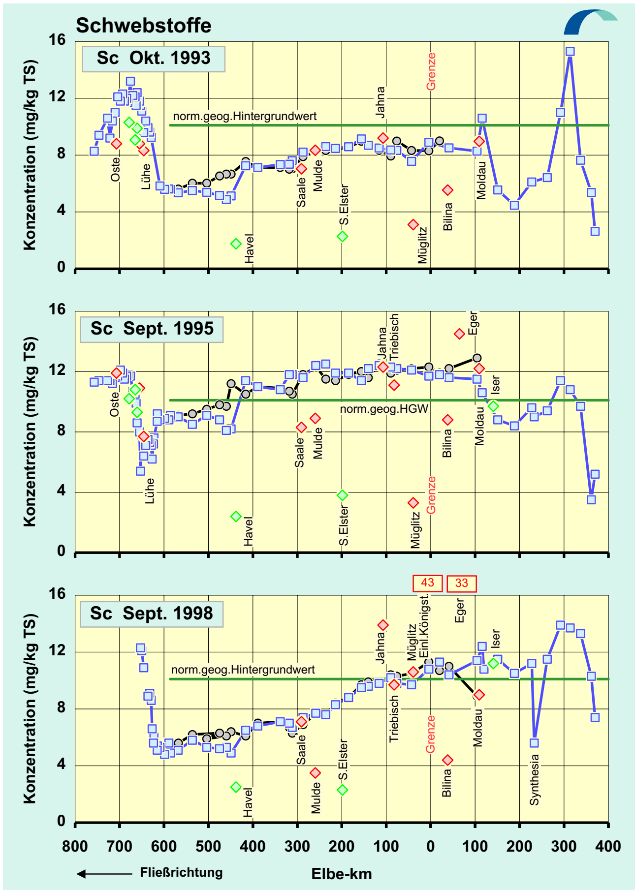
Abb.21c: Vergleich der Scandium -Konzentrationen in der Schwebstoff -Trockensubstanz (TS) der Elbe von der Mündung bis zur Quelle: Oktober 1993 / Sept. 1995 / Sept. 1998
