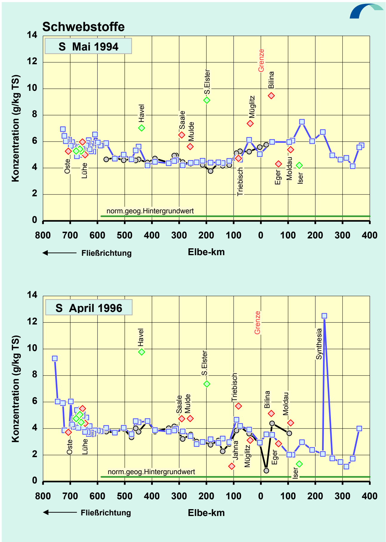
Abb.18d: Vergleich der Schwefel -Konzentrationen in der Schwebstoff -Trockensubstanz (TS) der Elbe von der Mündung bis zur Quelle: Mai 1994 / April 1996
