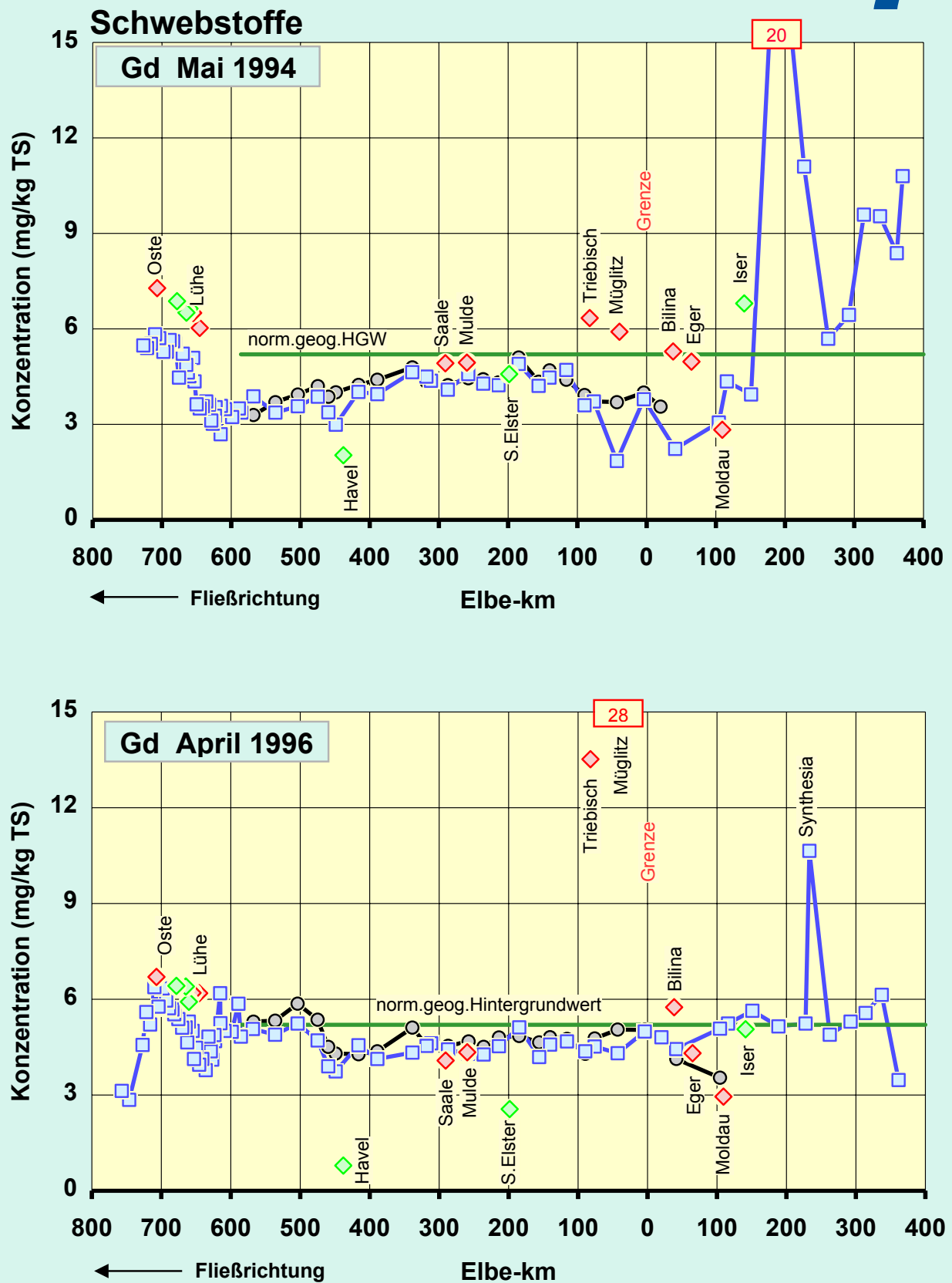
Abb.54d: Vergleich der Gadolinium -Konzentrationen in der Schwebstoff -Trockensubstanz (TS) der Elbe von der Mündung bis zur Quelle: Mai 1994 / April 1996
