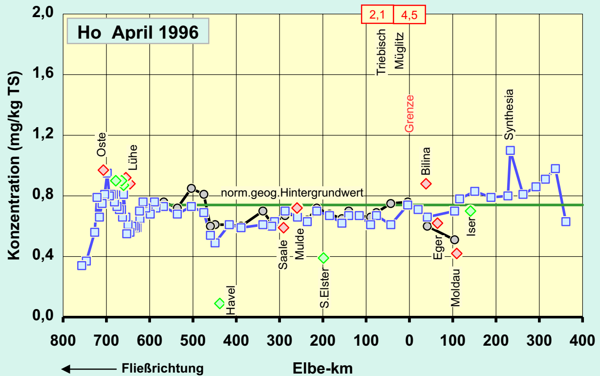
Abb.57d: Vergleich der Holmium -Konzentrationen in der Schwebstoff -Trockensubstanz (TS) der Elbe von der Mündung bis zur Quelle: Mai 1994 / April 1996
