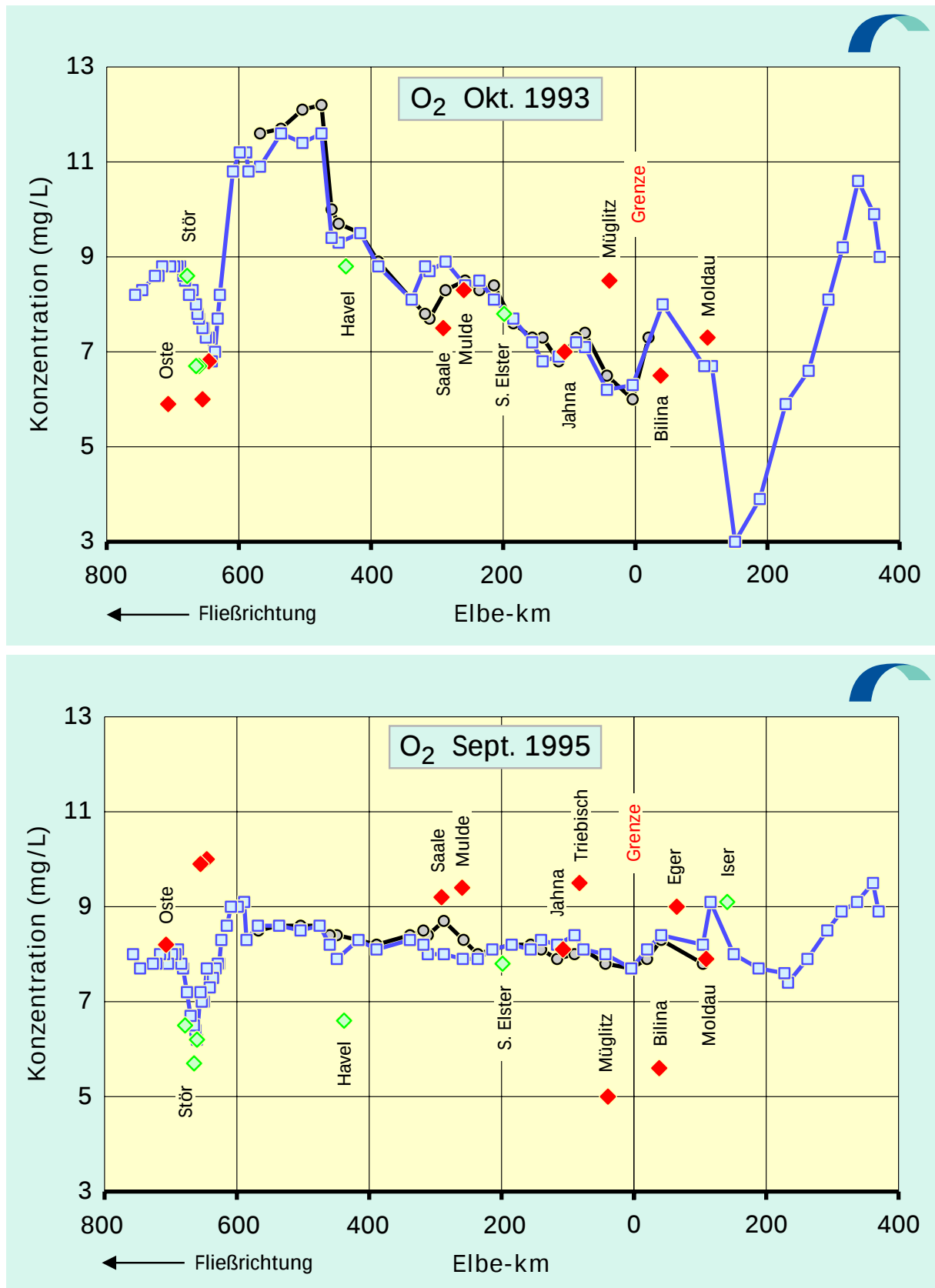
Abb. 4.5: Sauerstoff-Konzentrationen der Elbe von der Mündung bis zur Quelle: Oktober 1993 / September 1995
