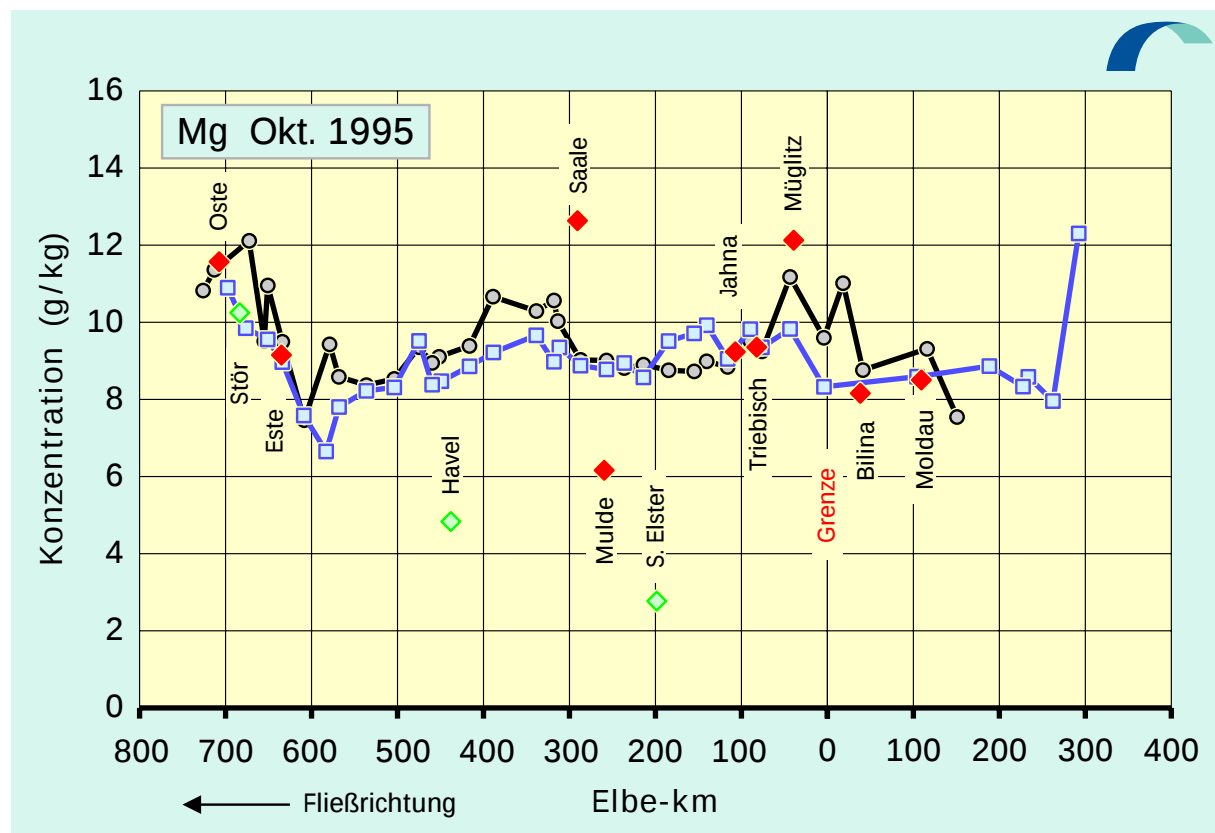
Abb. 4.37: Magnesium-Konzentrationen der Elbe-Sedimente (< 20 µm-Fraktion) von der Mündung bis zur Quelle: Oktober 1992 / Oktober 1995
