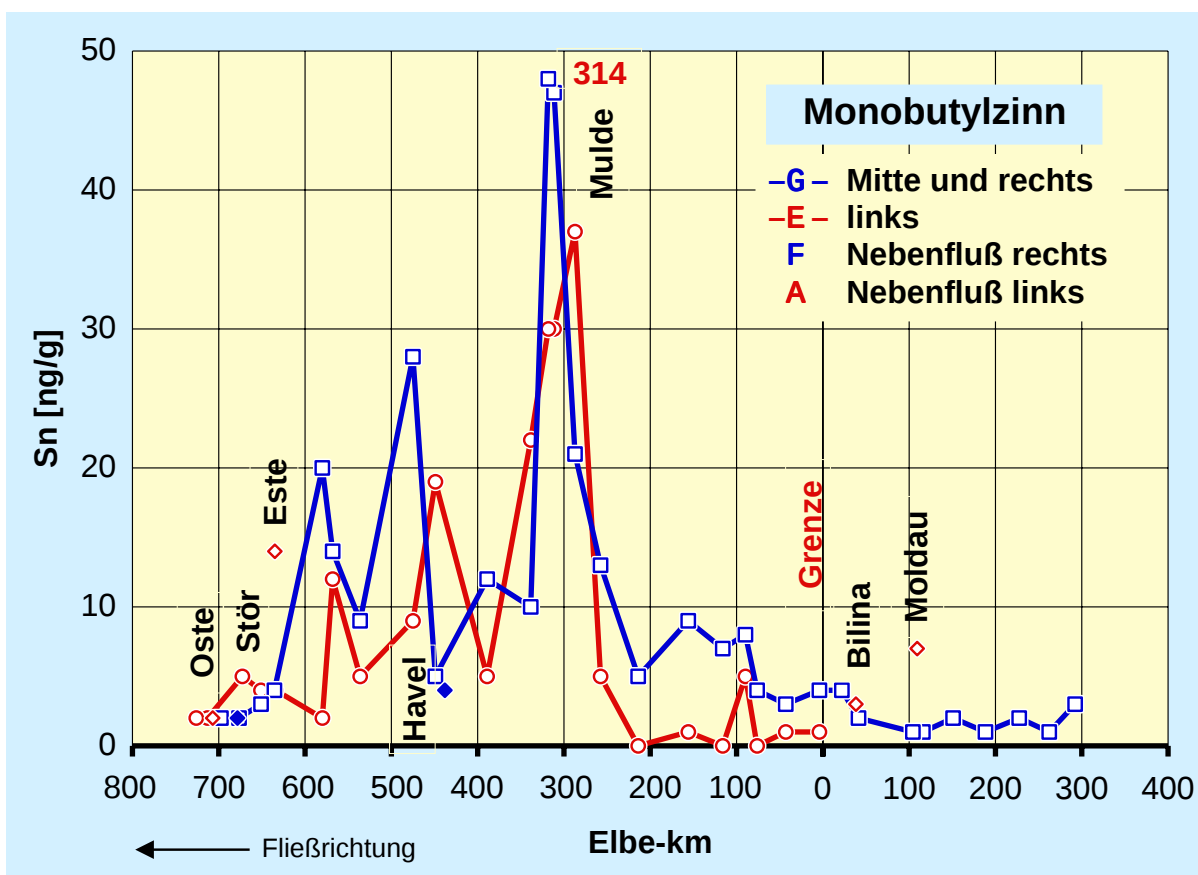
Abb. 4.77: Monobutylzinngelhalte in Oberflächensedimenten der Elbe: Längsprofil 1992
