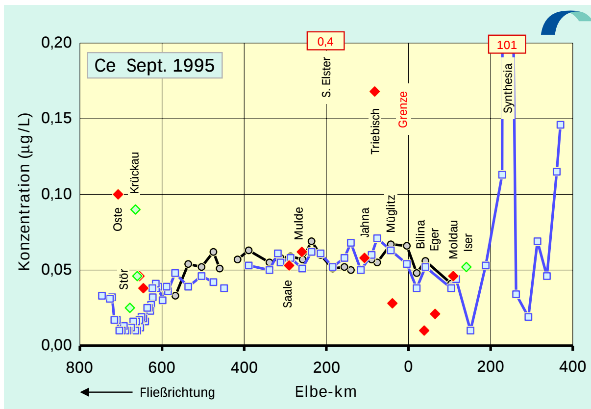
Abb. 4.19: Cer-Konzentrationen in Filtraten der Elbe von der Mündung bis zur Quelle: September 1995
