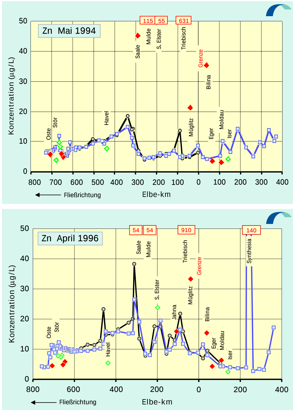
Abb. 4.13b: Zink-Konzentrationen in Filtraten der Elbe von der Mündung bis zur Quelle: Mai 1994 / April 1996
