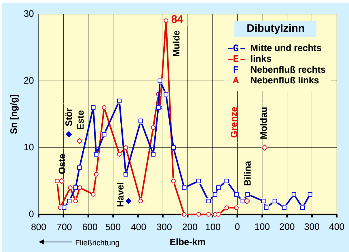
Abb. 4.76: Dibutylzinngelhalte in Oberflächensedimenten der Elbe: Längsprofil 1992
