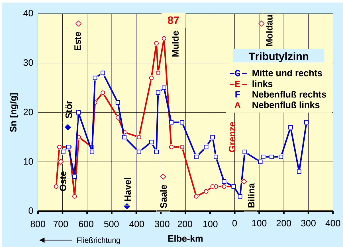
Abb. 4.75: Tributylzinngelhalte in Oberflächensedimenten der Elbe: Längsprofil 1992
