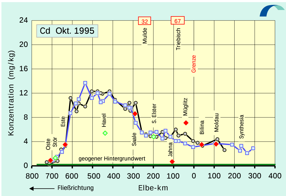
Abb. 4.40: Cadmium-Konzentrationen der Elbe-Sedimente (< 20 µm-Fraktion) von der Mündung bis zur Quelle: Oktober 1992 / Oktober 1995
