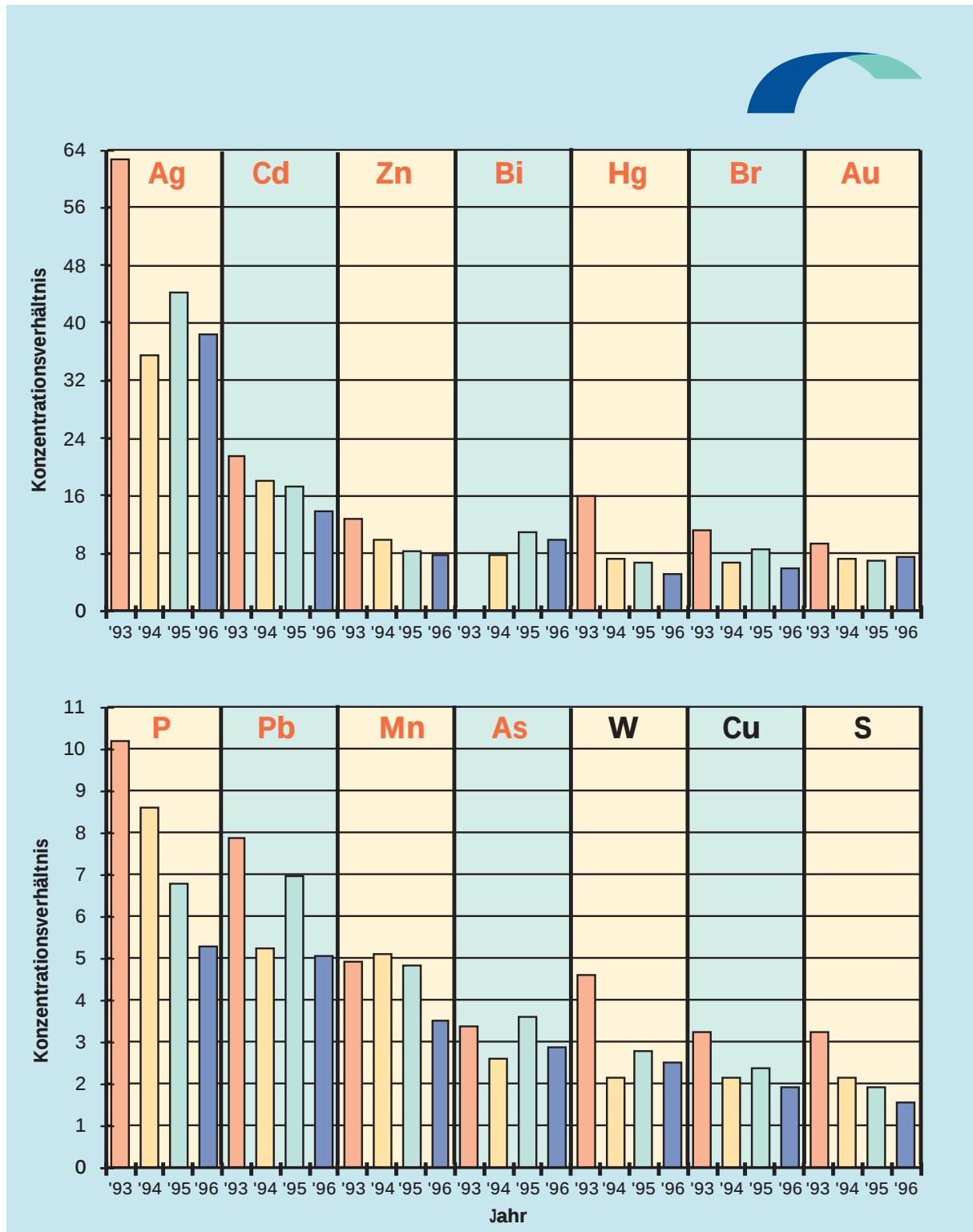
Abb. 6.3: Verhältnisse der Mediane der Elementkonzentrationen der Elbeschwebstoffe im Vergleich zum Internationalen Tongesteinstandard
