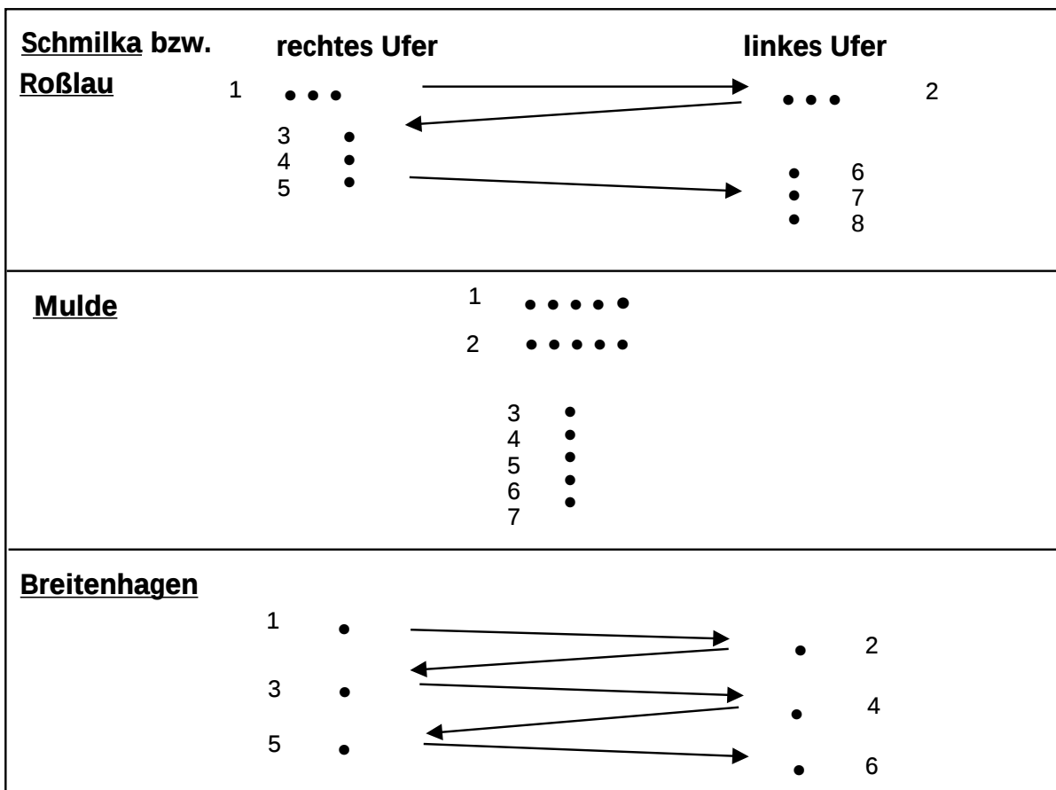
Abb. 3.5: Probennahmeplan für systematische Untersuchungen zur Schwebstoffprobennahme (• : Probennahme, nebeneinander: zeitgleich; untereinander: zeitlich versetzt)
