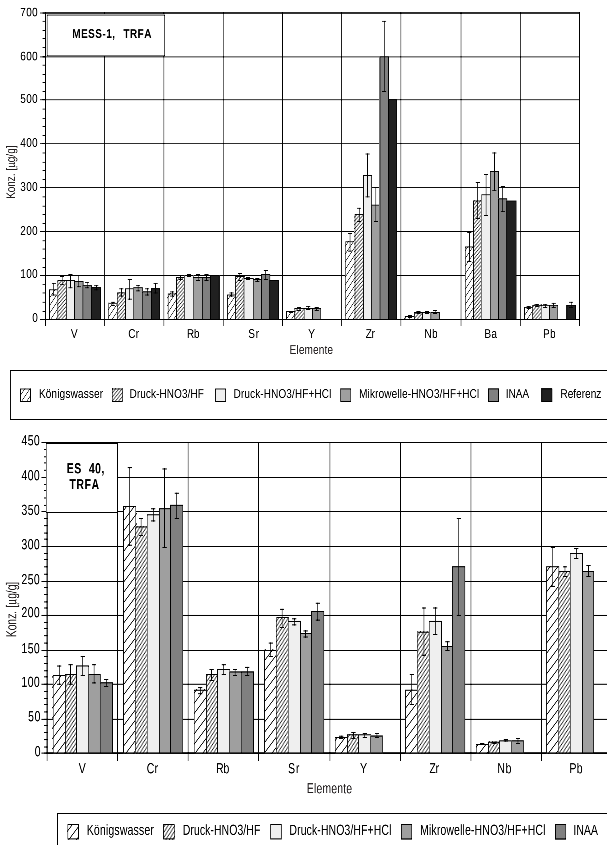
Abb. 3.16: Vergleich der TRFA-Ergebnisse verschiedener Aufschlußprozeduren mit Ergebnissen der INAA und Referenzwerten für Spurenelemente in MESS-1 und ES-40, Fehlerbalken: Standardabweichung der gesamten Prozedur (Aufschluß und Analyse)
