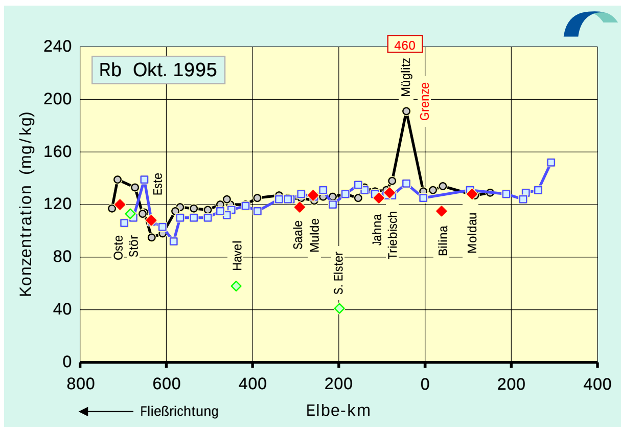
Abb. 4.35: Rubidium-Konzentrationen der Elbe-Sedimente (< 20 \mu m-Fraktion) von der Mündung bis zur Quelle: Oktober 1992 / Oktober 1995
