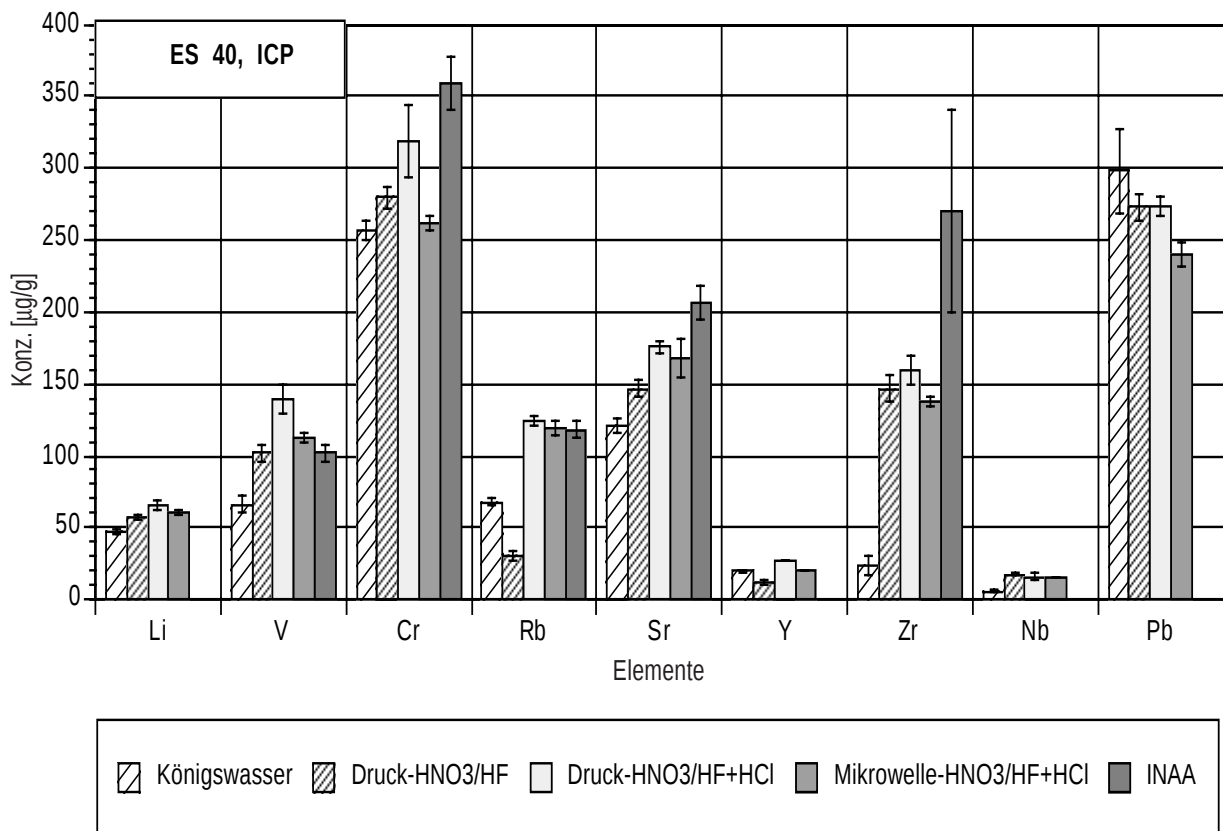
Abb. 3.15: Vergleich der ICP-Ergebnisse verschiedener Aufschlußprozeduren mit Ergebnissen der INAA für Hauptkomponenten und Spurenelemente in ES 40, Fehlerbalken: Standardabweichung der gesamten Prozedur (Aufschluß und Analyse)
