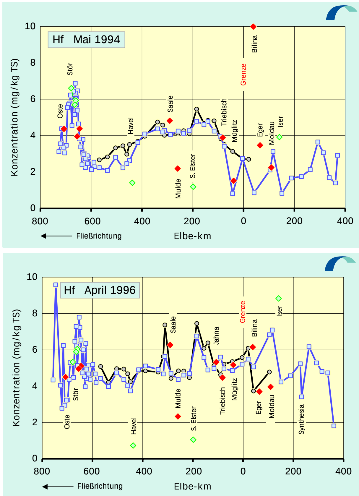
Abb. 4.21: Hafnium-Konzentrationen in der Schwebstoff-Trockensubstanz (TS) der Elbe von der Mündung bis zur Quelle: Mai 1994 / April 1996
