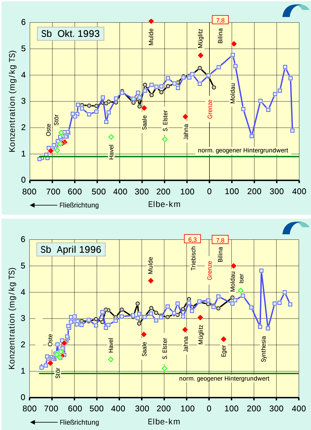
Abb. 4.26: Antimon-Konzentrationen in der Schwebstoff-Trockensubstanz (TS) der Elbe von der Mündung bis zur Quelle: Oktober 1993 / April 1996
