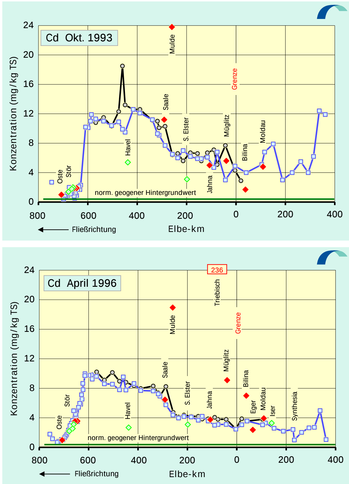
Abb. 4.31: Cadmium-Konzentrationen in der Schwebstoff-Trockensubstanz (TS) der Elbe von der Mündung bis zur Quelle: Oktober 1993 / April 1996
