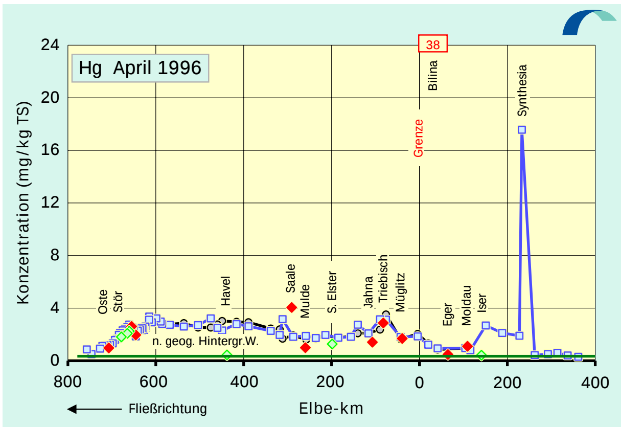
Abb.4.23b: Quecksilber-Konzentrationen in der Schwebstoff-Trockensubstanz (TS) der Elbe von der Mündung bis zur Quelle: Mai 1994 / April 1996
