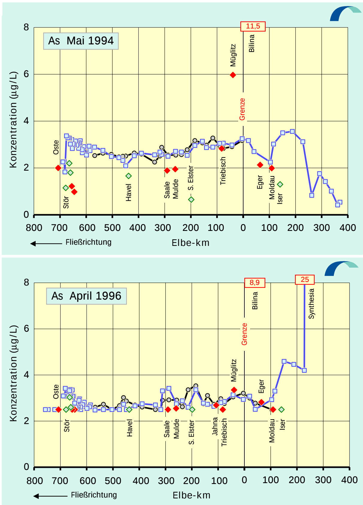
Abb. 4.16b: Arsen-Konzentrationen in Filtraten der Elbe von der Mündung bis zur Quelle: Mai 1994 / April 1996
