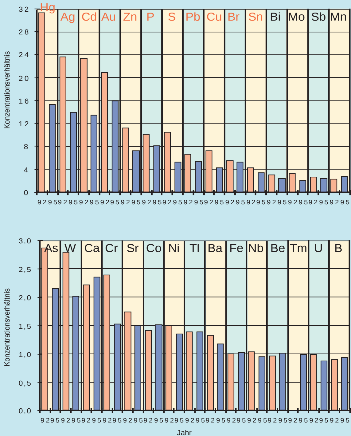
Abb. 6.4: Verhältnisse der Mediane der Elementkonzentrationen in den Elbsedimenten im Vergleich zu den elbspezifischen geogenen Hintergrundwerten
