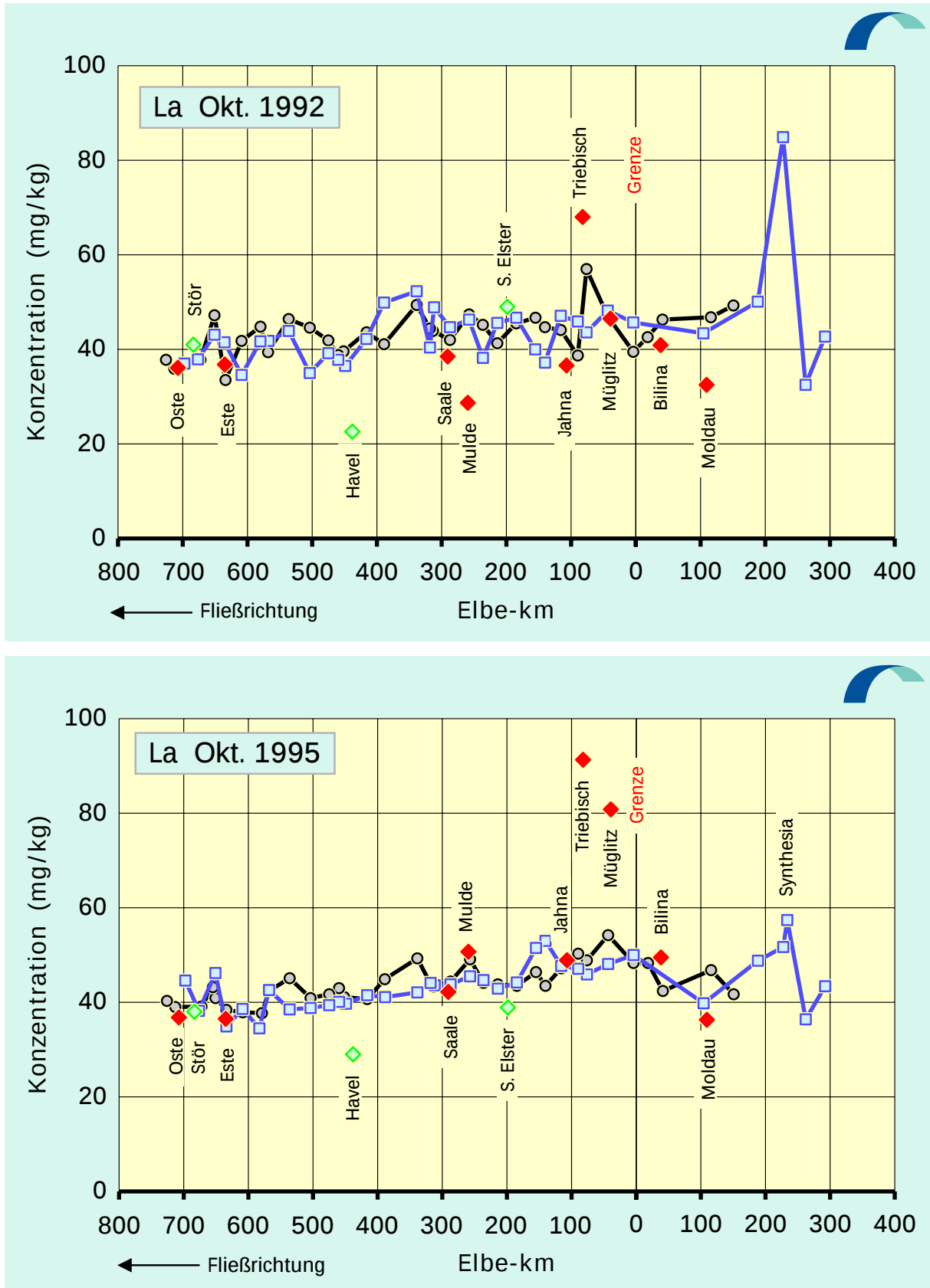
Abb. 4.36: Lanthan-Konzentrationen der Elbe-Sedimente (< 20 µm-Fraktion) von der Mündung bis zur Quelle: Oktober 1992 / Oktober 1995
