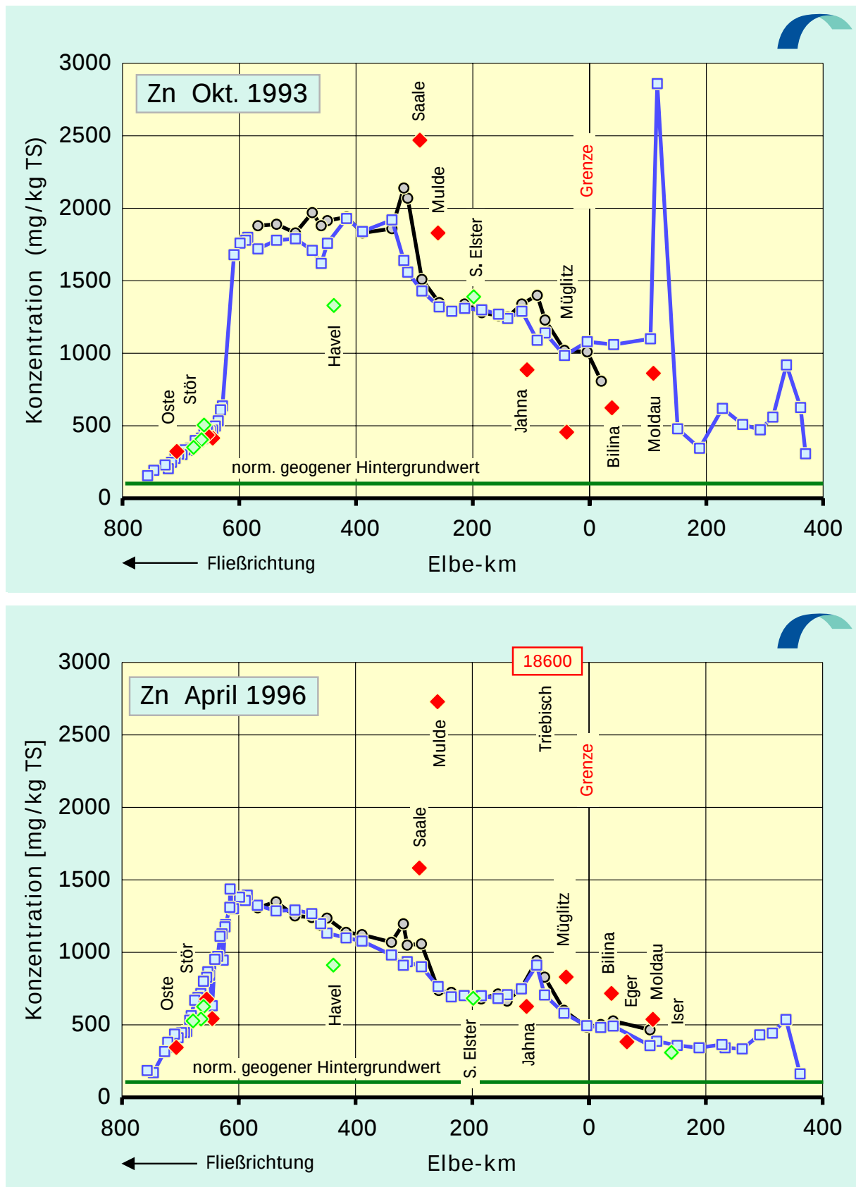
Abb. 4.30: Zink-Konzentrationen in der Schwebstoff-Trockensubstanz (TS) der Elbe von der Mündung bis zur Quelle: Oktober 1993 / April 1996
