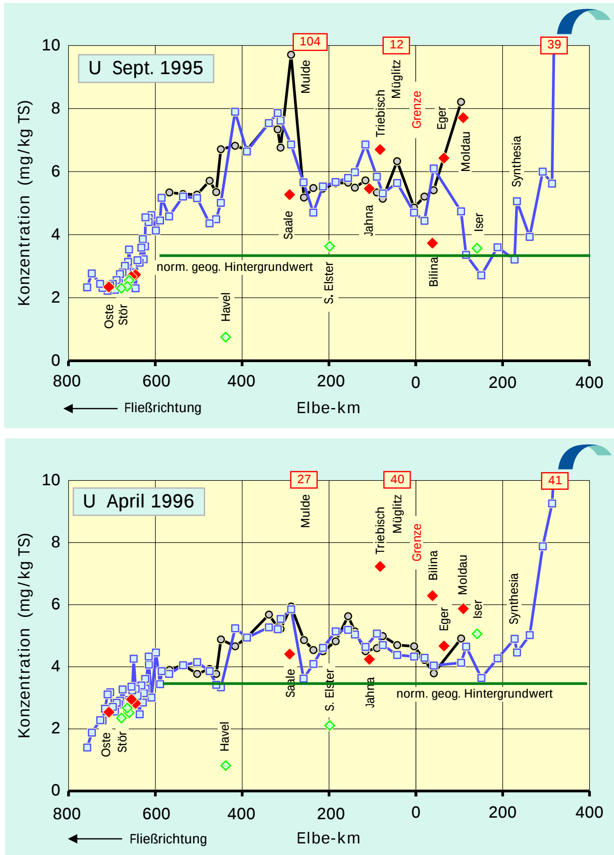
Abb. 4.24b: Uran-Konzentrationen in der Schwebstoff-Trockensubstanz (TS) der Elbe von der Mündung bis zur Quelle: September 1995 / April 1996
