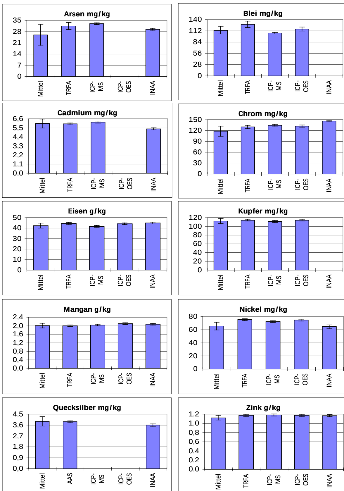
Abb. 3.23: Ergebnisse der Ringanalyse von schwebstoffbütigem Sediment (29 Labore) (Landesamt für Umweltschutz Sachsen-Anhalt, 1995)
