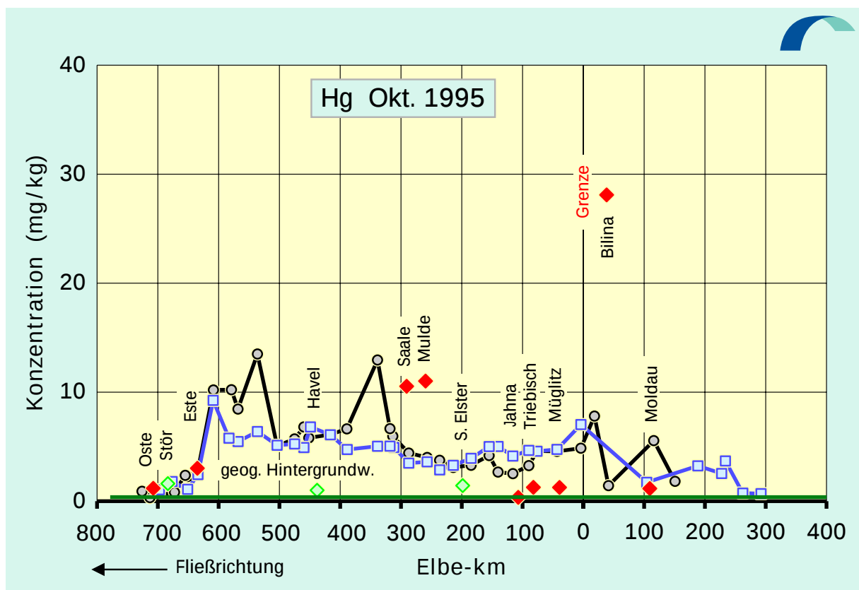
Abb. 4.38: Quecksilber-Konzentrationen der Elbe-Sedimente (< 20 µm-Fraktion) von der Mündung bis zur Quelle: Oktober 1992 / Oktober 1995
