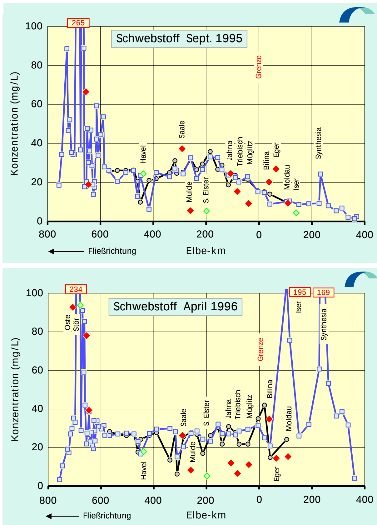
Abb. 4.4: Schwebstoff-Konzentrationen der Elbe von der Mündung bis zur Quelle: September 1995 / April 1996
