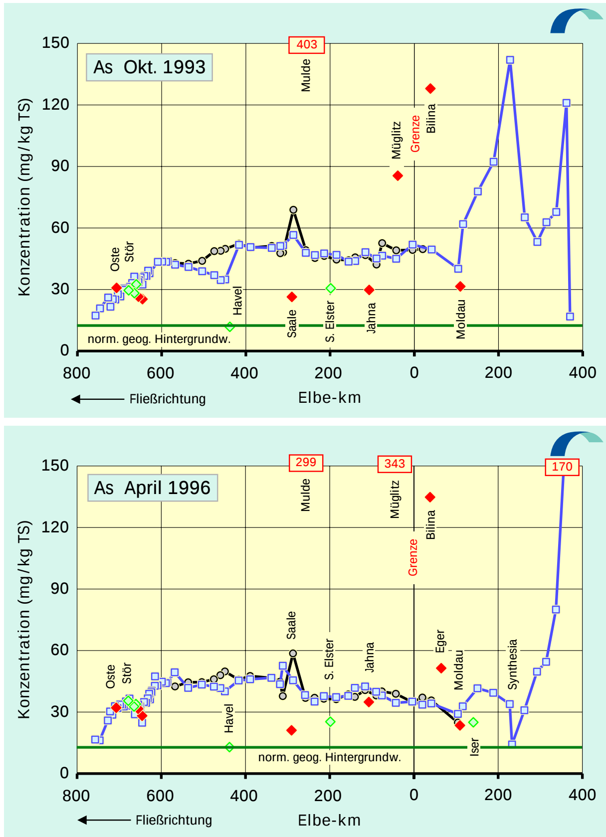
Abb. 4.28: Arsen-Konzentrationen in der Schwebstoff-Trockensubstanz (TS) der Elbe von der Mündung bis zur Quelle: Oktober 1993 / April 1996
