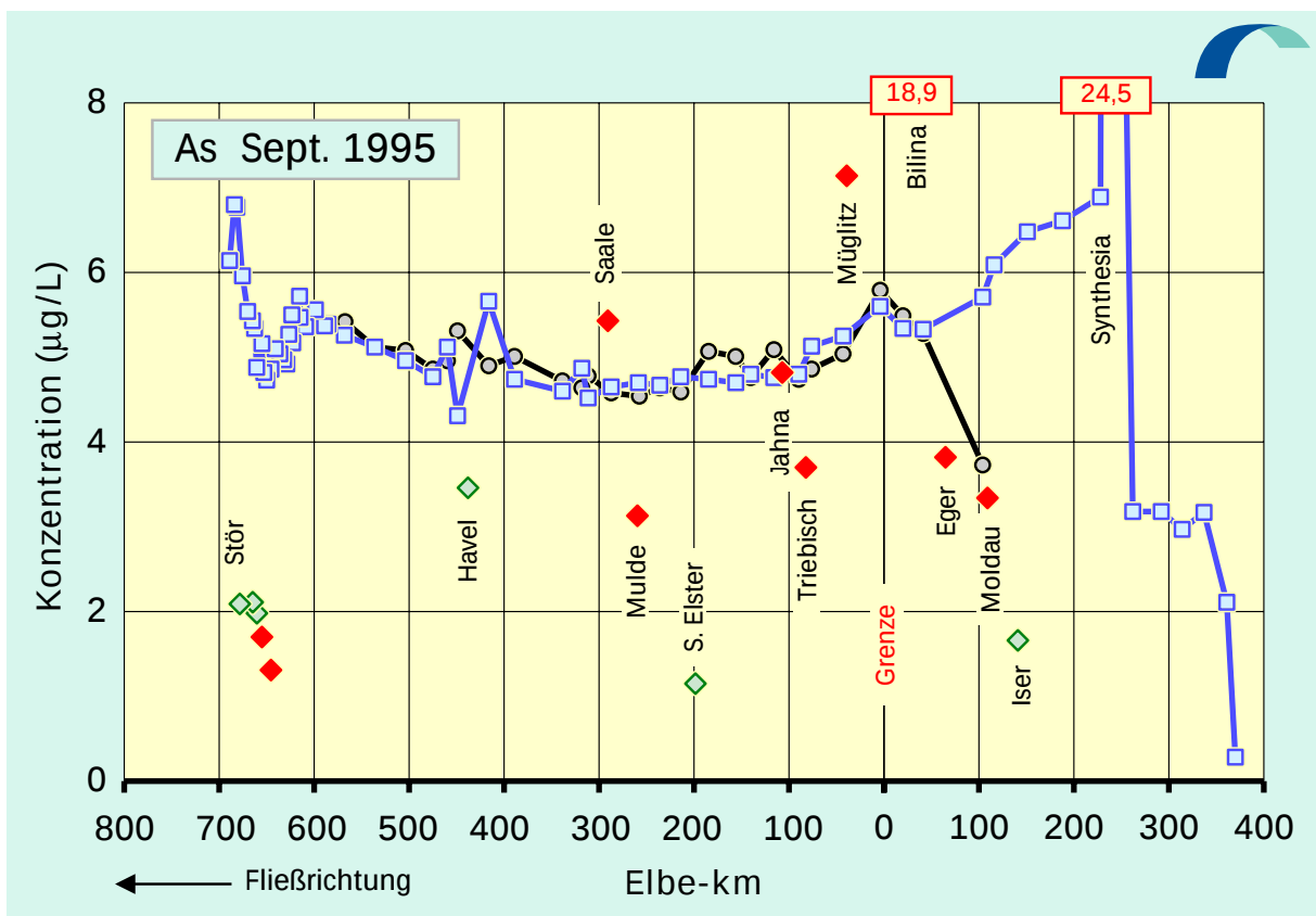
Abb. 4.16a: Arsen-Konzentrationen in Filtraten der Elbe von der Mündung bis zur Quelle: Oktober 1993 / September 1995
