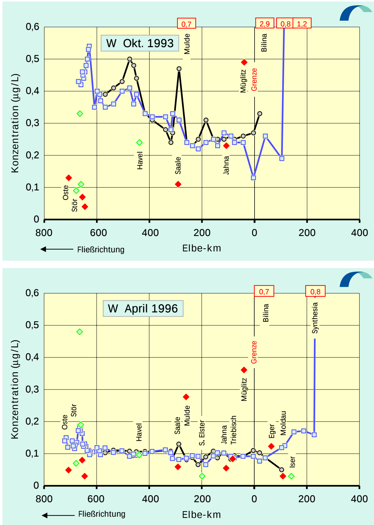
Abb. 4.18: Wolfram-Konzentrationen in Filtraten der Elbe von der Mündung bis zur Quelle: Oktober 1993 / April 1996
