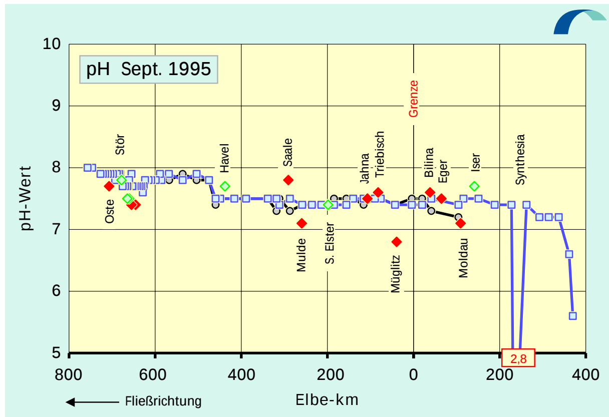
Abb. 4.2: pH-Werte der Elbe von der Mündung bis zur Quelle:
