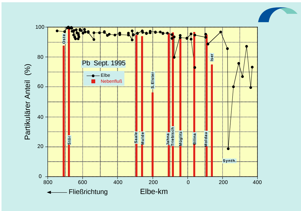
Abb. 4.57: Prozentuale partikuläre Anteile von Titan und Blei (1995)
