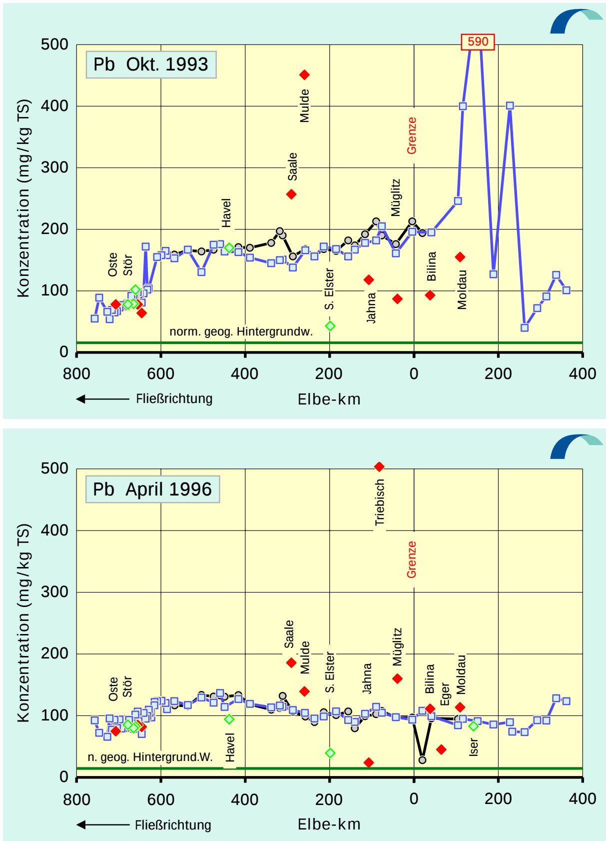
Abb. 4.29: Blei-Konzentrationen in der Schwebstoff-Trockensubstanz (TS) der Elbe von der Mündung bis zur Quelle: Oktober 1993 / April 1996
