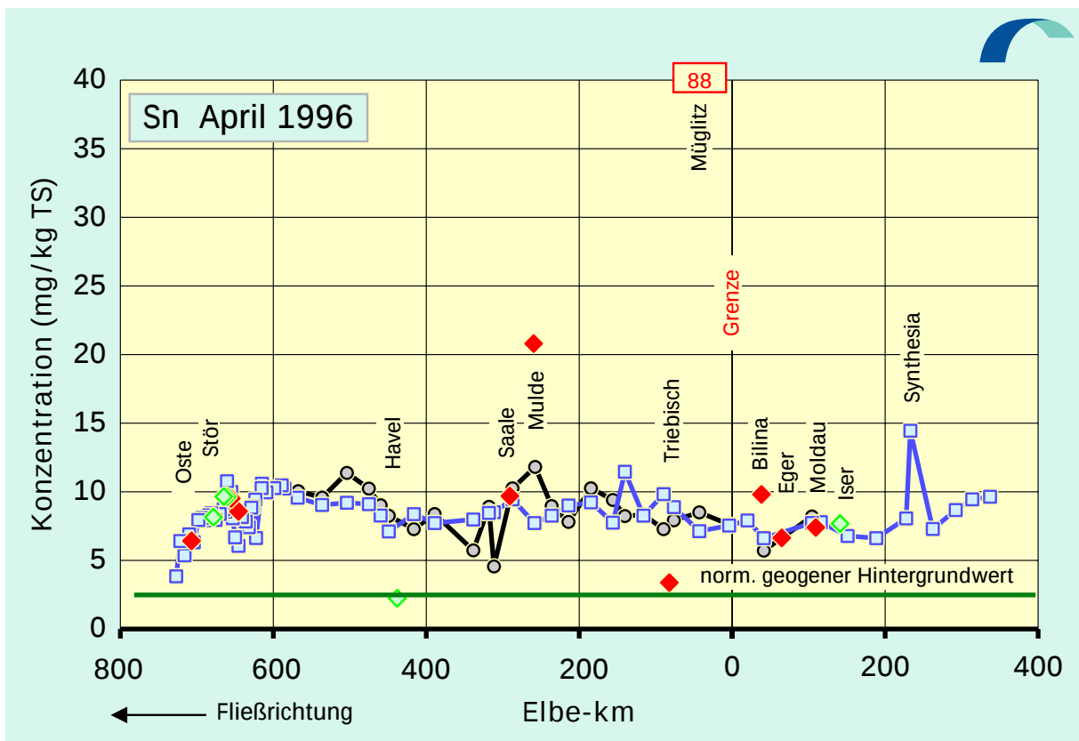
Abb. 4.32: Zinn-Konzentrationen in der Schwebstoff-Trockensubstanz (TS) der Elbe von der Mündung bis zur Quelle: Oktober 1993 / April 1996
