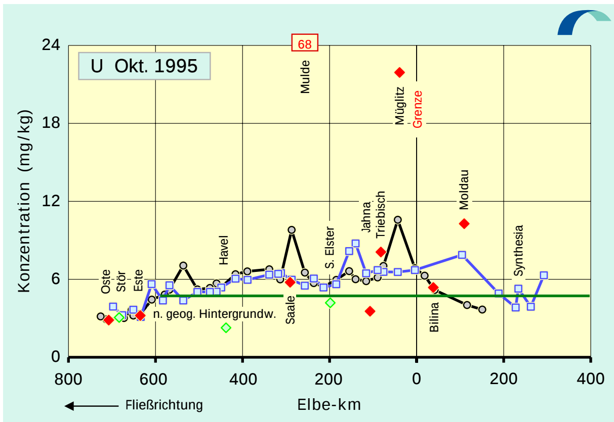
Abb. 4.41: Uran-Konzentrationen der Elbe-Sedimente (< 20 \mu m-Fraktion) von der Mündung bis zur Quelle: Oktober 1992 / Oktober 1995
