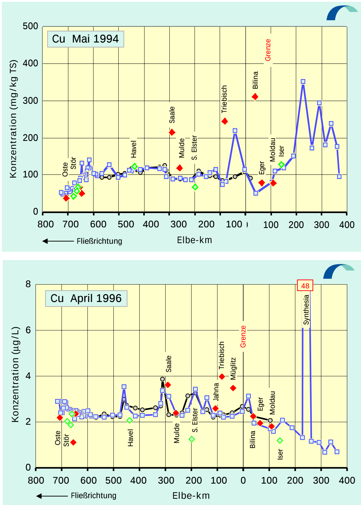
Abb. 4.12: Kupfer-Konzentrationen in Filtraten der Elbe von der Mündung bis zur Quelle: Mai 1994 / April 1996
