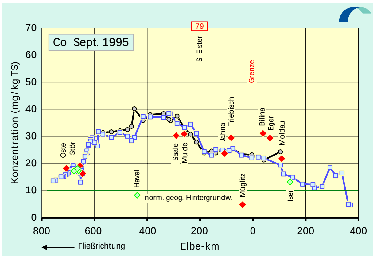
Abb. 4.33: Cobalt-Konzentrationen in der Schwebstoff-Trockensubstanz (TS) der Elbe von der Mündung bis zur Quelle: Oktober 1993 / September 1995
